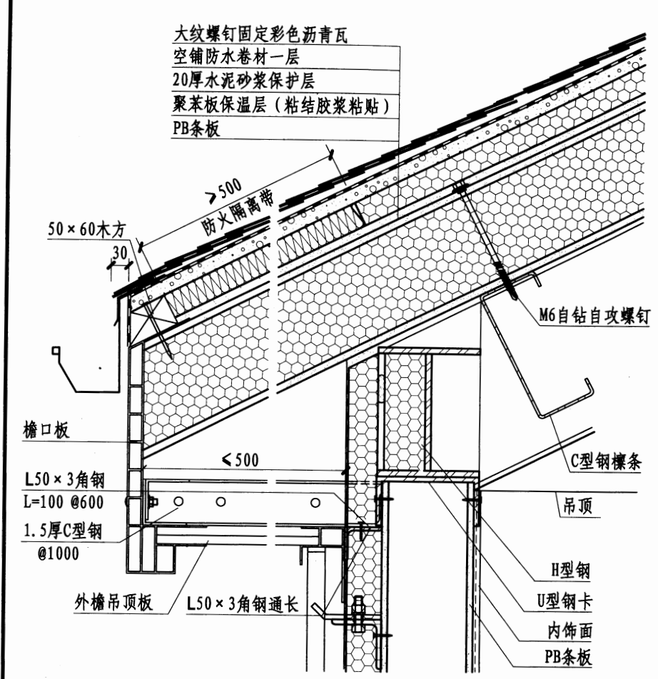
① 彩色沥青瓦屋面
