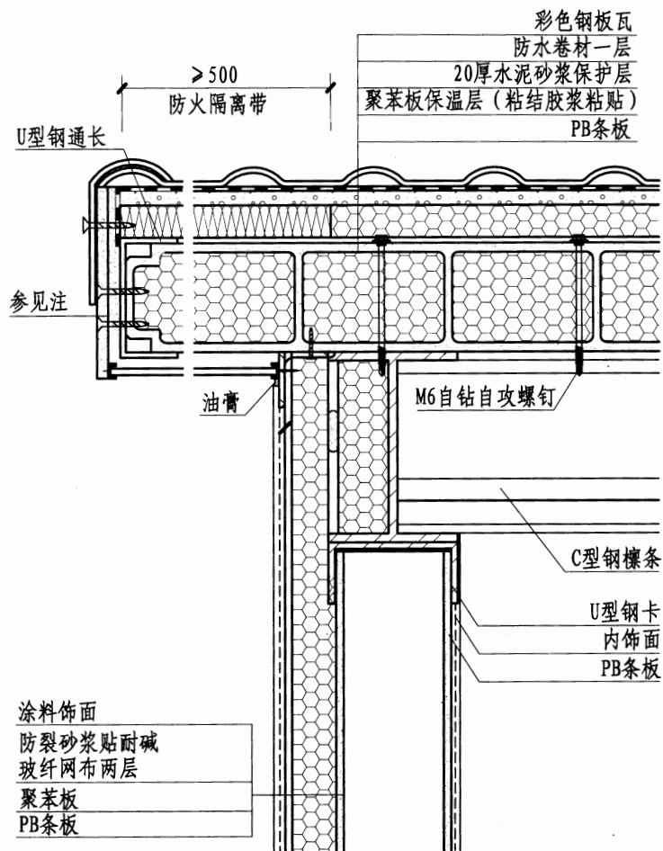
② 彩钢瓦屋面
