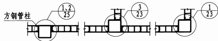
1-1与方型钢柱连接
