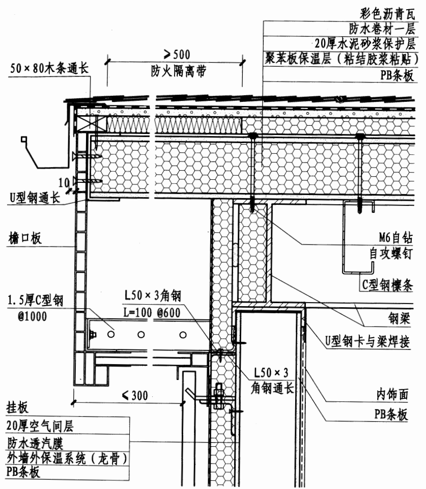
② 彩色沥青瓦屋面
