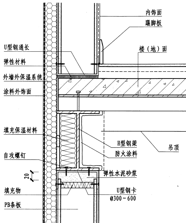
① 楼板与钢梁连接
