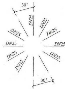
图 4.5.13 管径（压力）的标注位置示例
