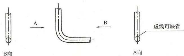
图 4.6.2 双线管道转向的画法
