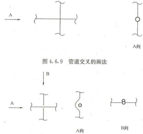
图 4.6.10 管道跨越的画法
