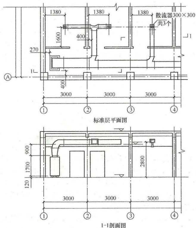
图 4.2.3 平、剖面示例
