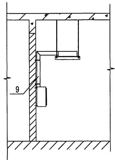
A-A 剖面图
