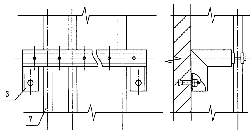
3 支架安装
