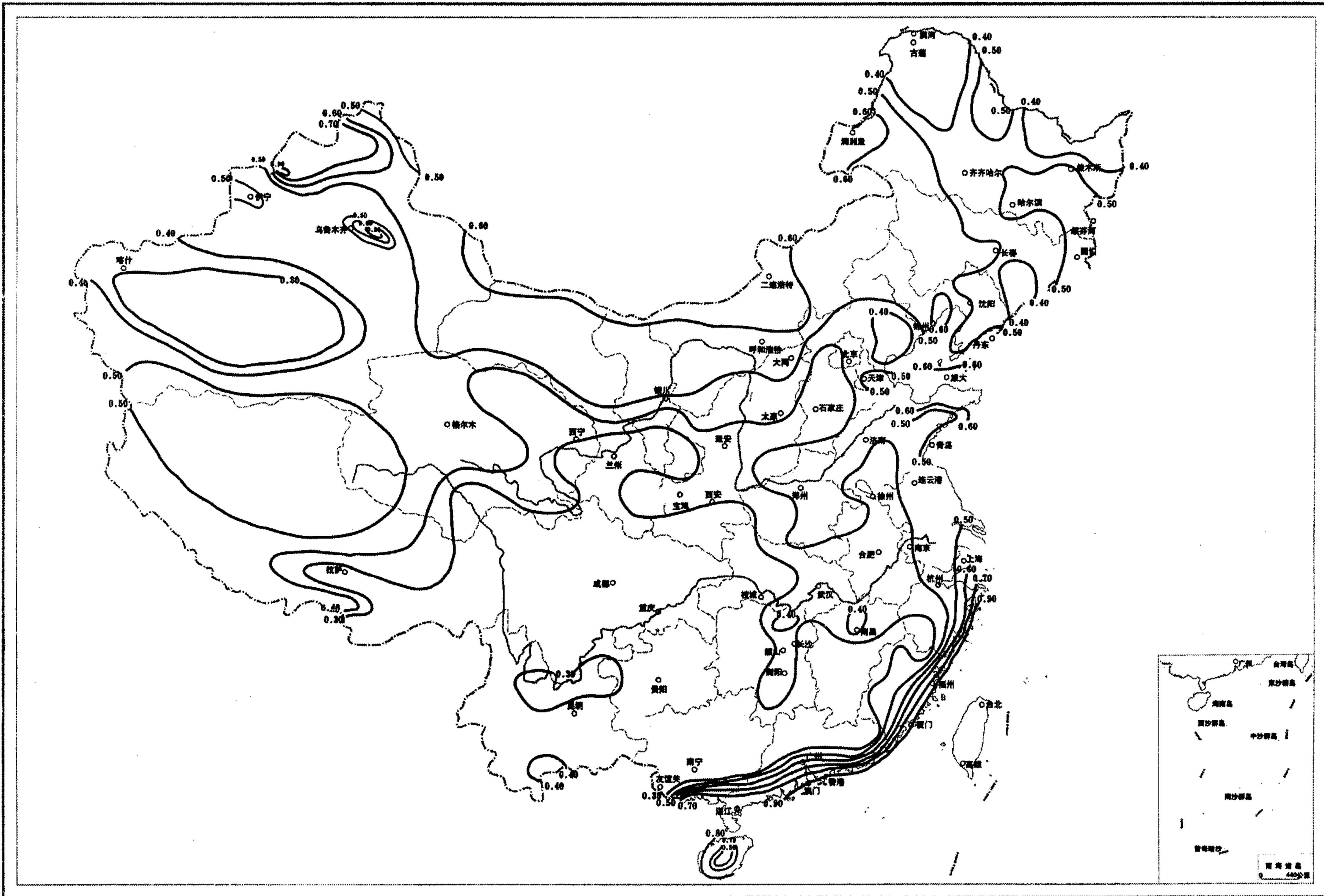
图1 全国基本风压分布图(单位: \text{KN/m}^2 )
