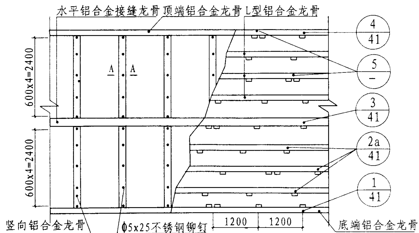
墙板、龙骨、支座布置图B(粘胶法)
