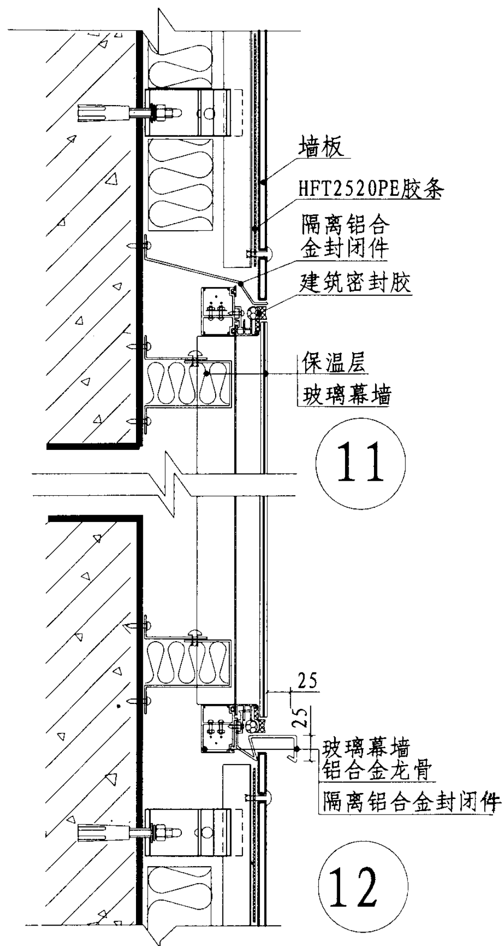
GL1与玻璃幕墙连接
