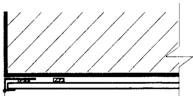
末端铝合金龙骨
