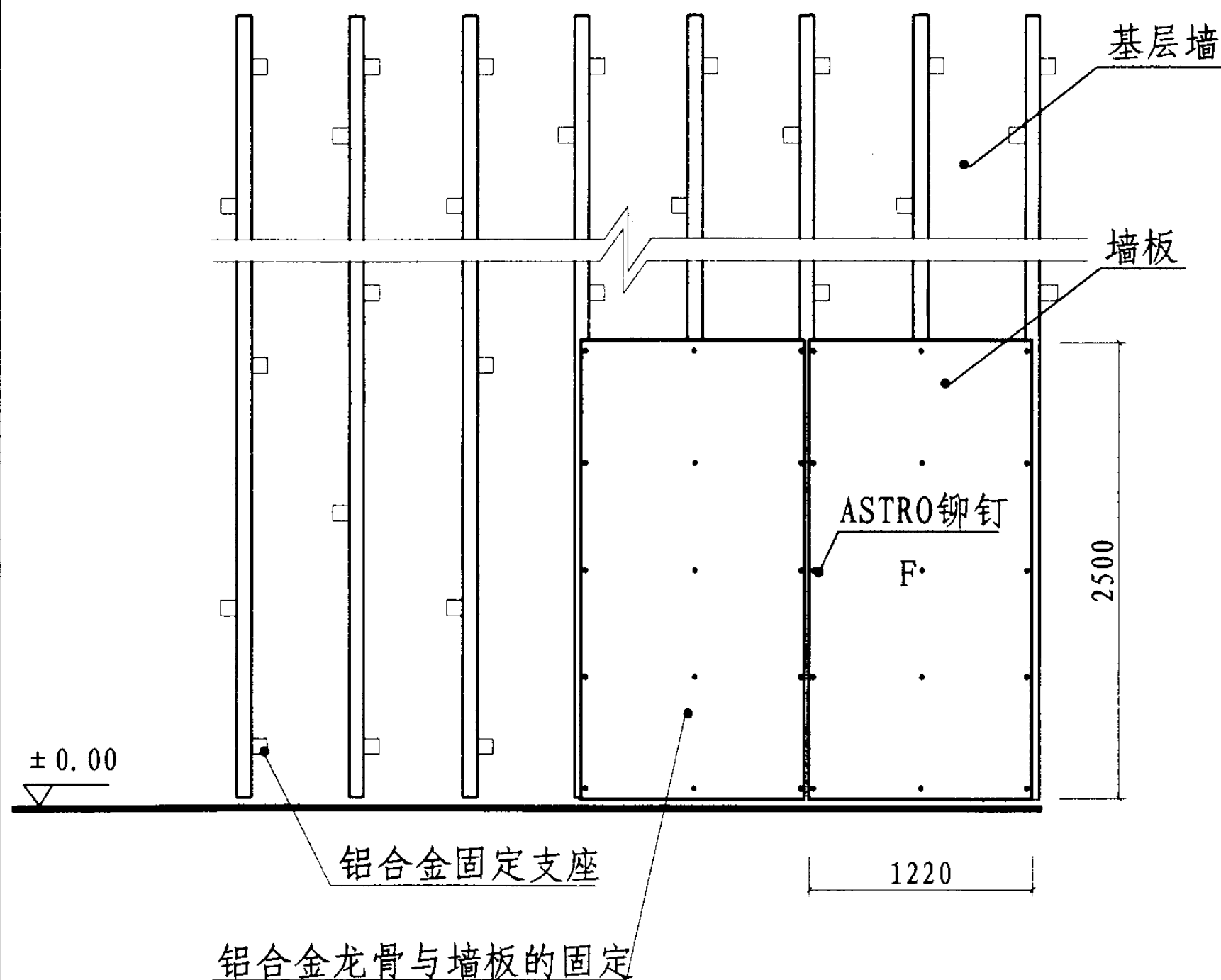
铝合金龙骨与墙板布置示意图
