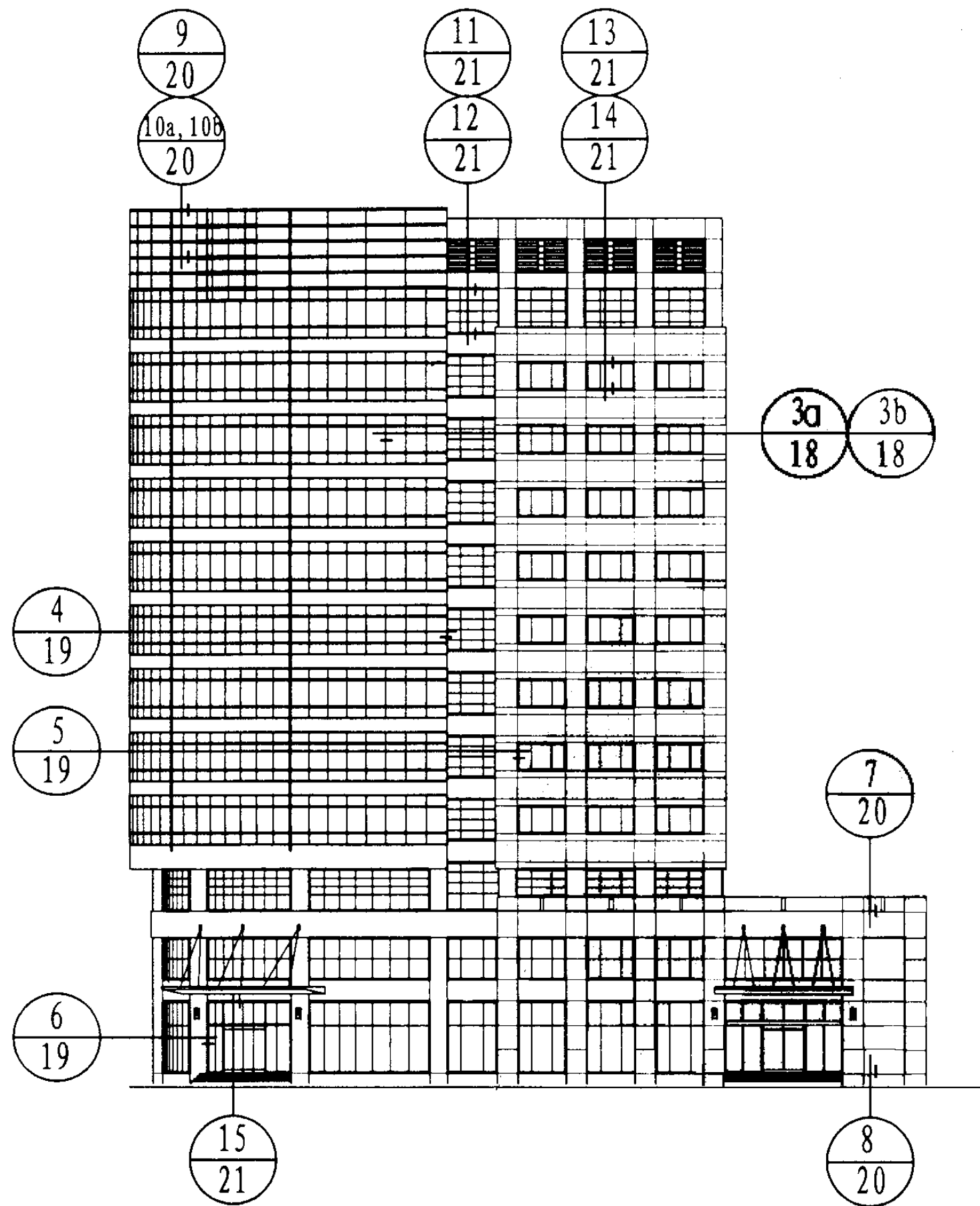
立面图
