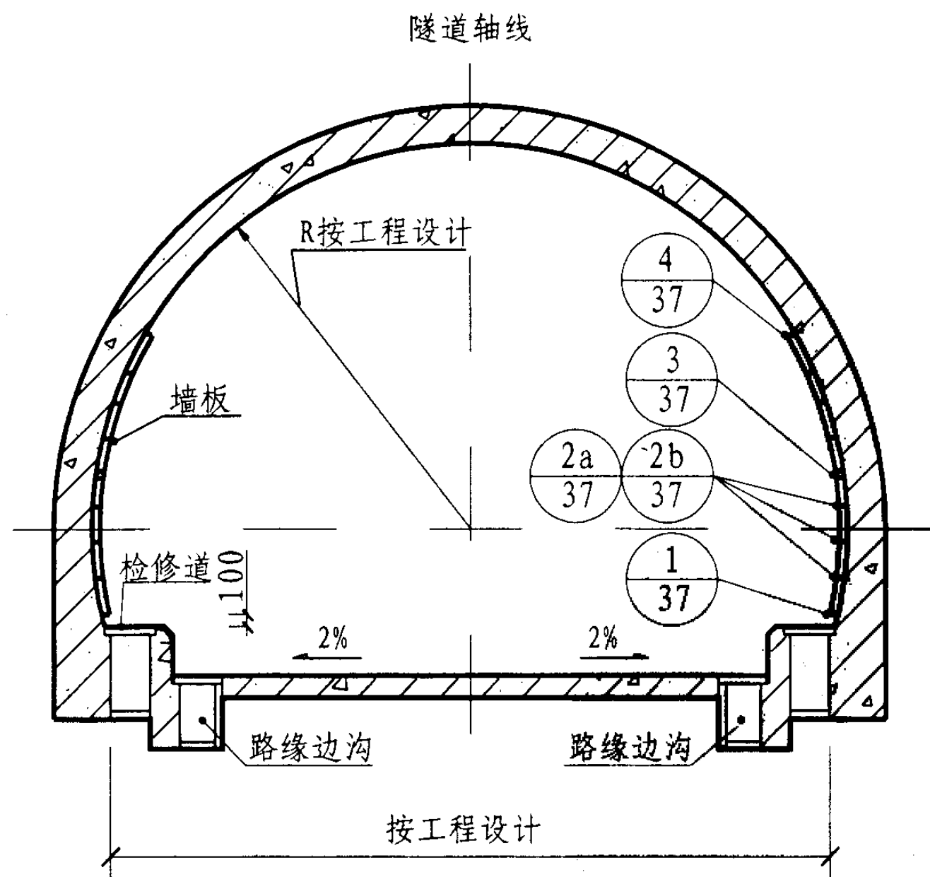
弧形隧道标准段剖面图（一）
