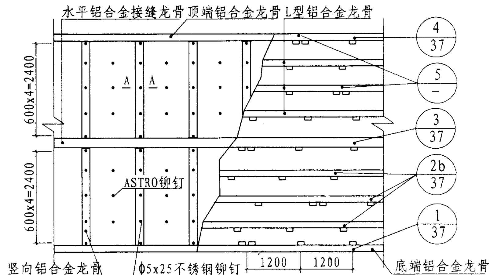
墙板、龙骨、支座布置图A(铆钉法)
