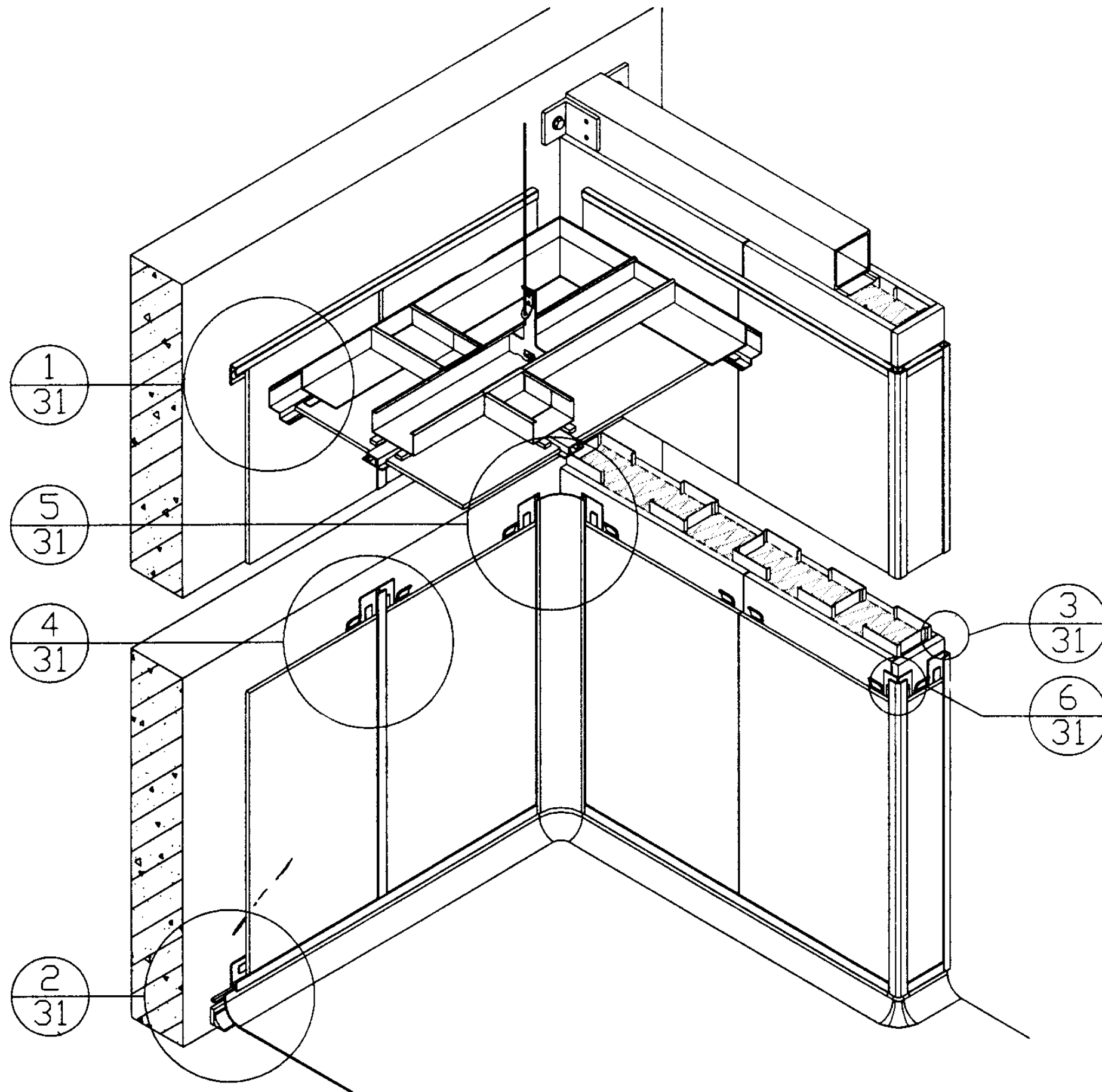
内墙GL3、GL4 索引图
