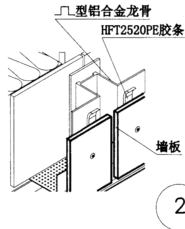
外墙GL2 铆钉固定法及详图 (一)
