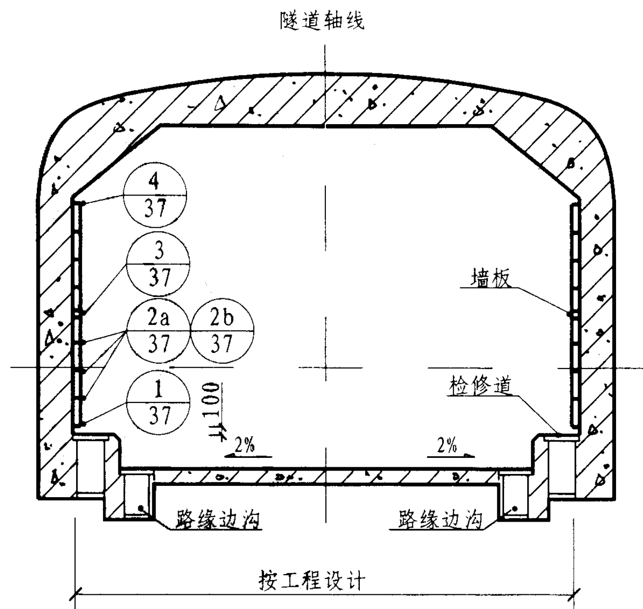
矩形隧道标准段剖面图（二）
