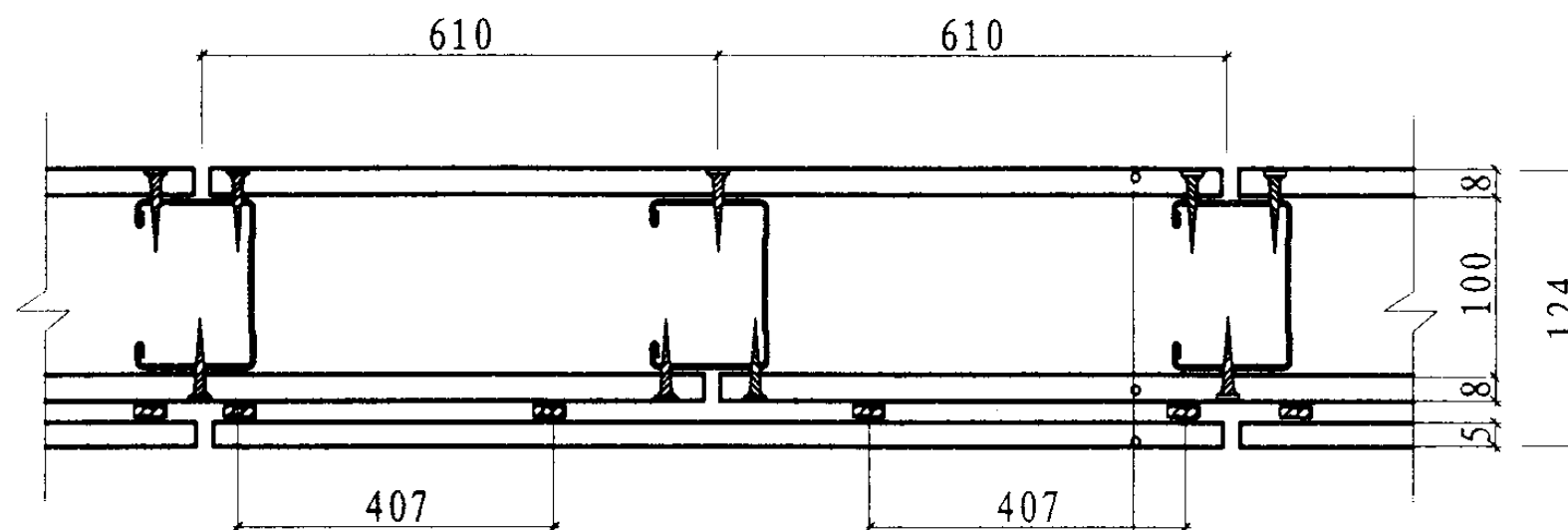
内墙 GL4a平面
