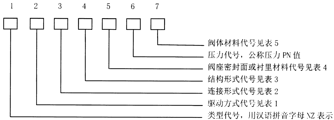
图2 铸石耐磨闸阀型号的单位组成
