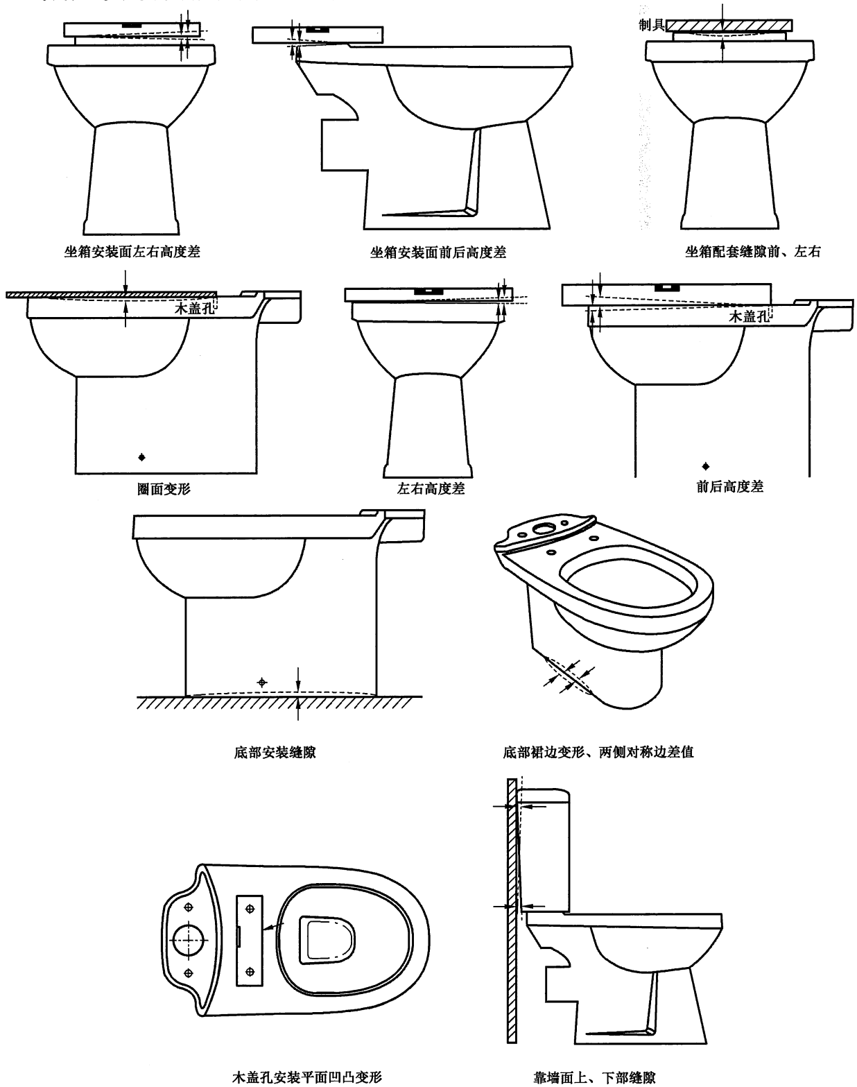
图 C.2 分体坐便器
