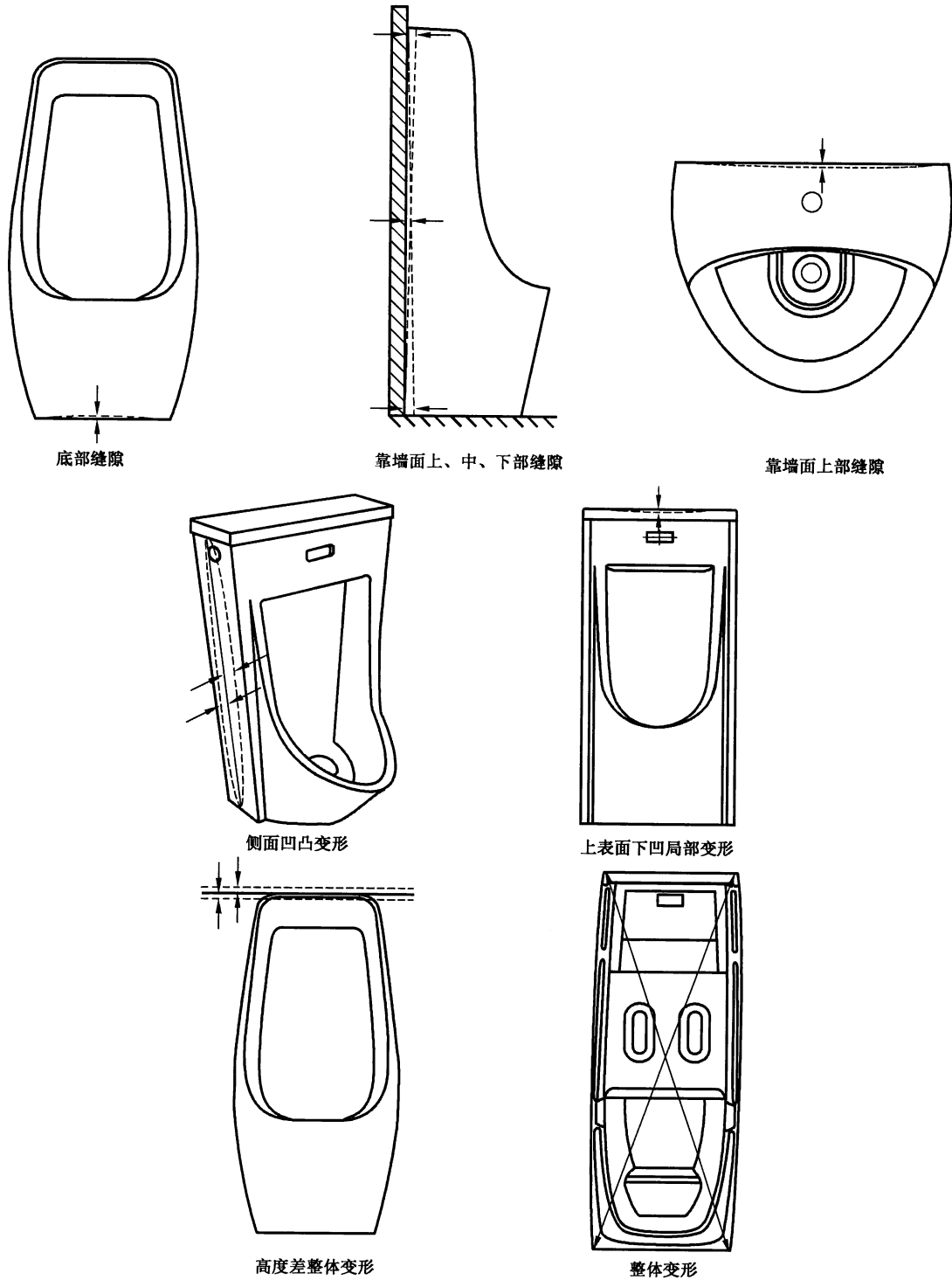
图 C.8 落地式小便器
