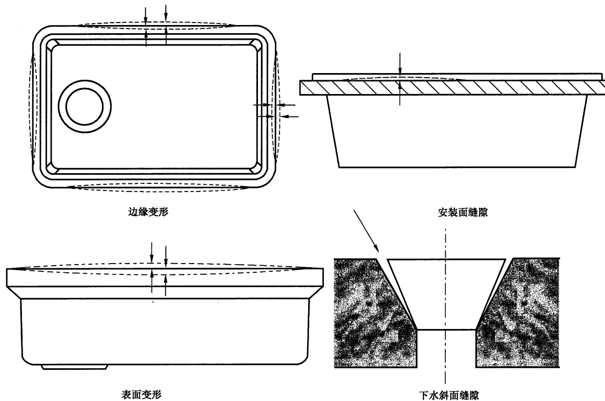
图 C.10 洗涤槽
