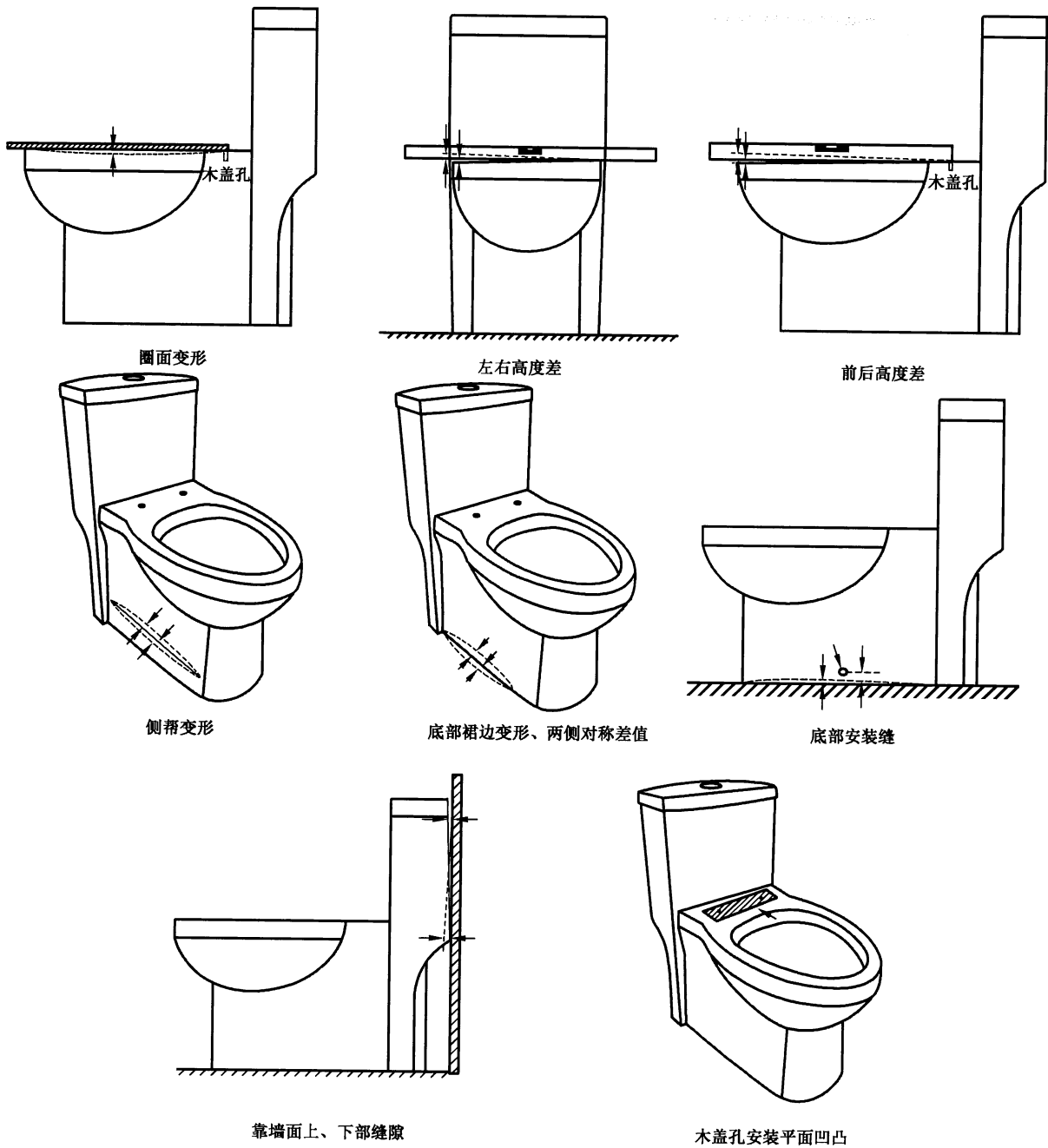
图 C.1 连体坐便器
