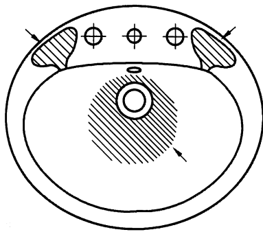
皂盒、洗净面不能存水
