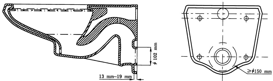
b) 壁挂式坐便器排污口尺寸
