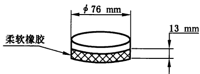
a) 洗涤槽试验板
