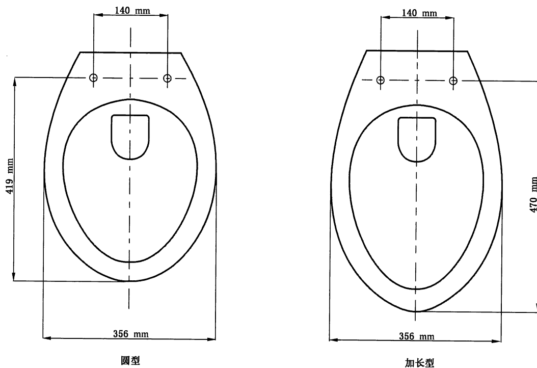
图 B.4 坐便器坐圈尺寸示意图
