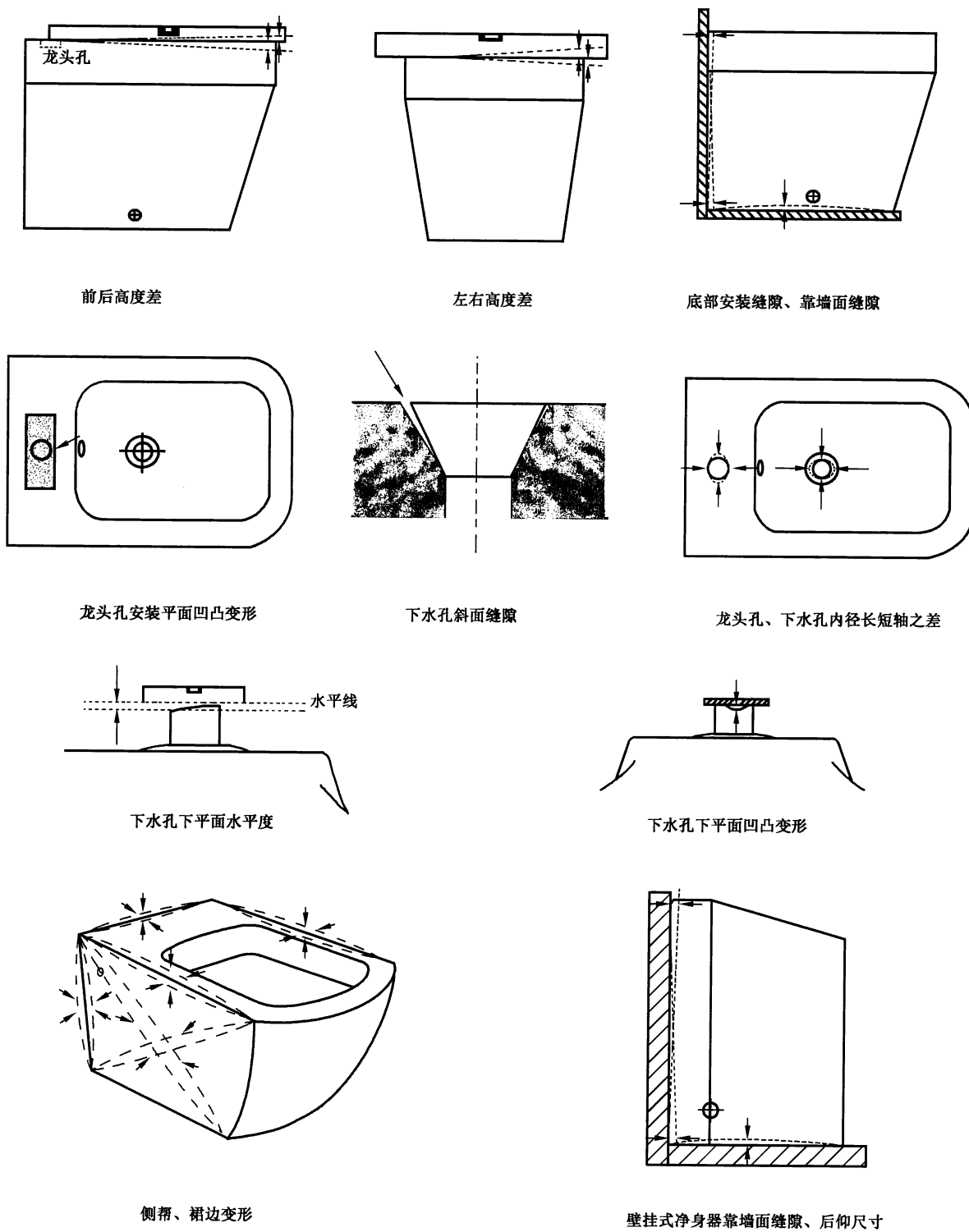
图 C.6 净身器
