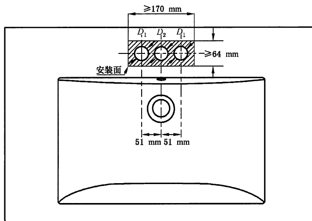
4寸孔图示
