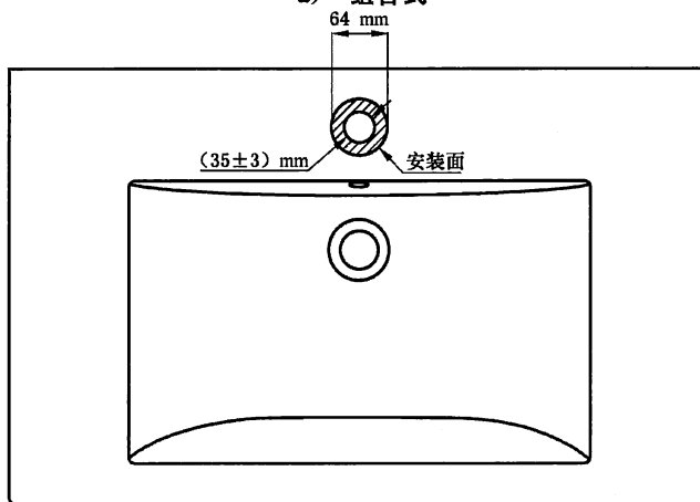
4寸孔图示
