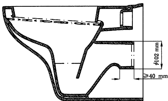
a) 下排式坐便器排污口尺寸
