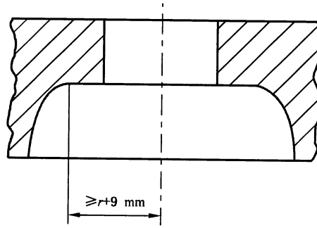
c) 洗面器背面安装平台
