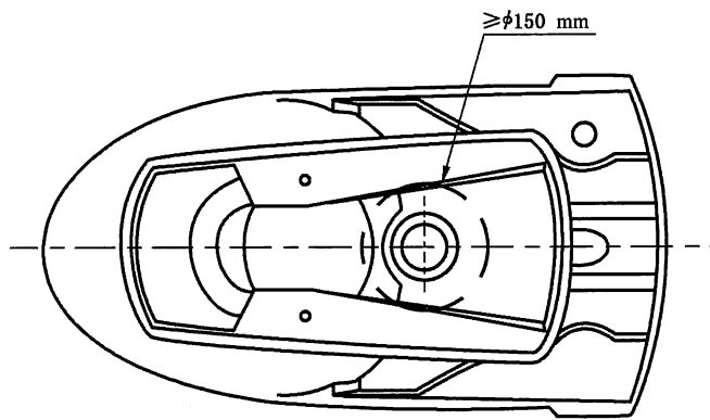
a) 下排式坐便器排污口尺寸
