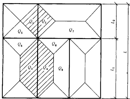
a) 若 L_2/L_1 < 1/2 且 X < L/3 时 则按下图计算:
