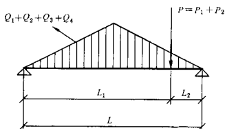
a) 若 L_2/L_1 < 1/2 且 X < L/3 时 则按下图计算:
