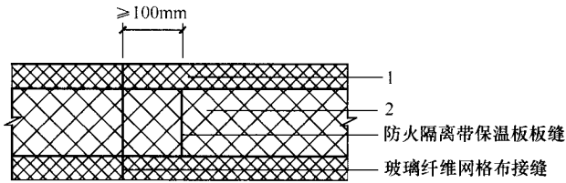
图 5.0.7-2 防火隔离带网格布水平方向对接
