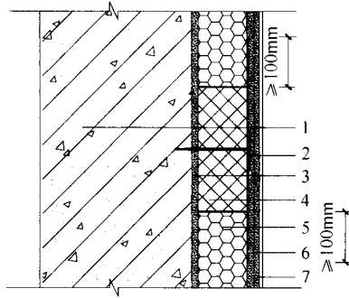
图 5.0.7-1 防火隔离带网格布垂直方向搭接
