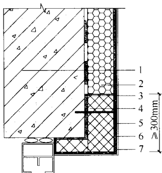
图 5.0.10 门窗洞口上部防火 隔离带做法（二）
