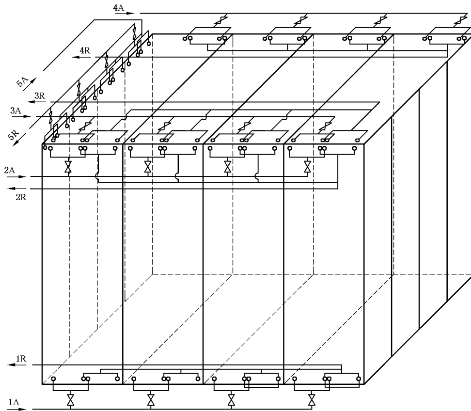
a) 水冷夹层水道接管示意图
