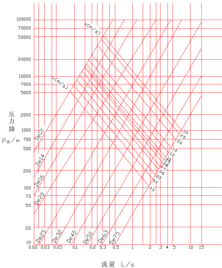
图 A.0.3 热水管水力计算图表
