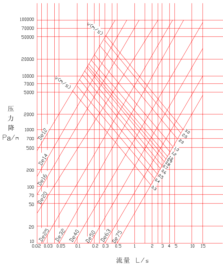
图 A.0.2 冷水管水力计算图表
