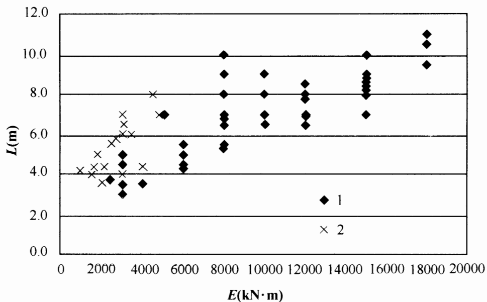
图 2 强夯置换主夯击能级与置换墩长度实测值关系图
