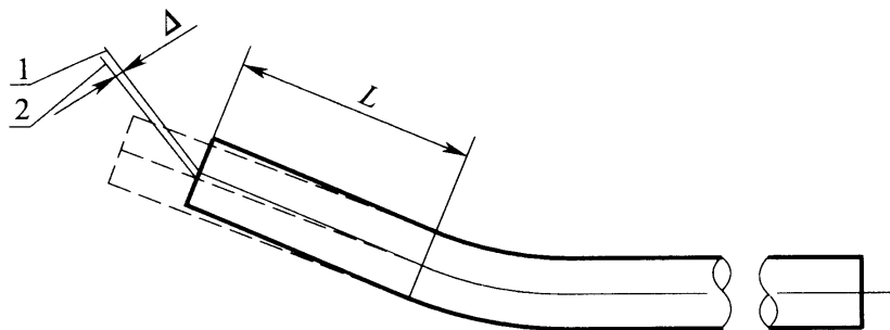
图 4.2.9 弯曲角度及管端中心偏差
