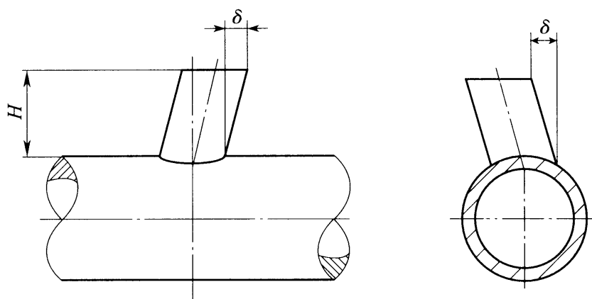
图 5.0.15-2 三通支管垂直度偏差 \delta
