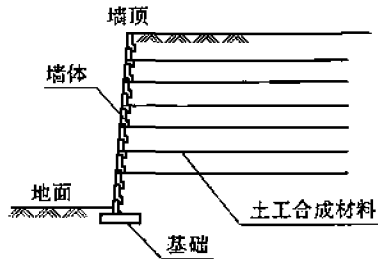
图 4 加筋式挡渣墙结构示意图
