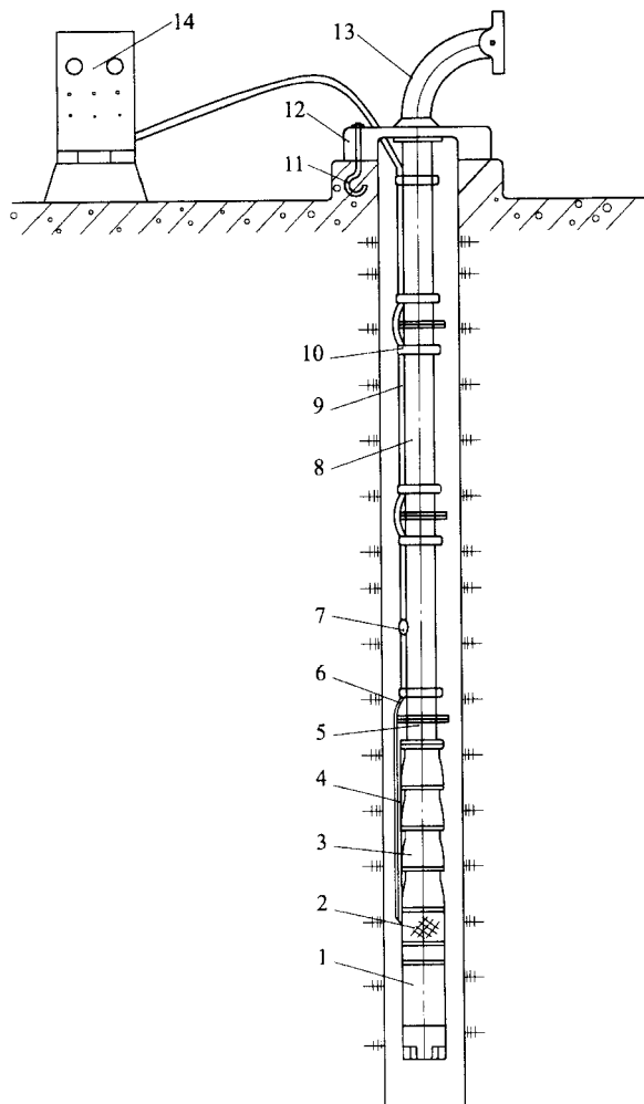
图 4.3.3 井用潜水泵安装
