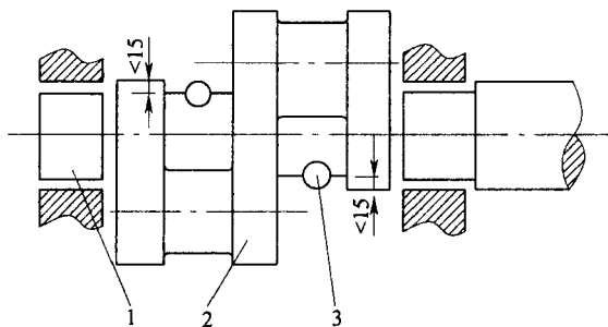
图 3.3.3-2 测量曲柄间距离
