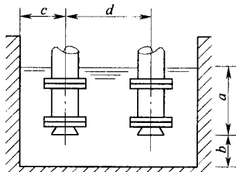
图 C.0.2-2 吸入池尺寸
