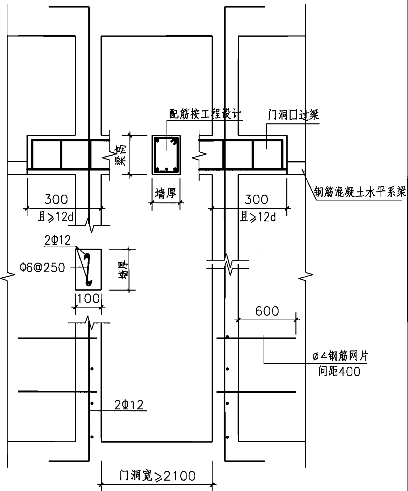
洞口抱框做法二
