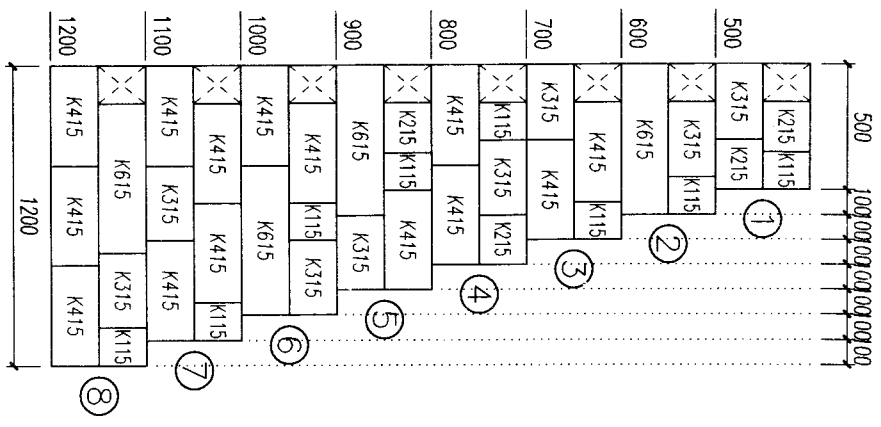
L形墙体砌法
