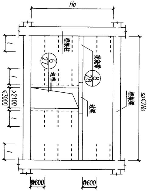
① 用于2.1m < 洞口宽度 ≤ 3.0m
