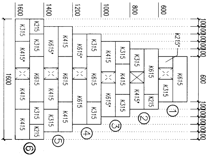
丁形墙体砌法
