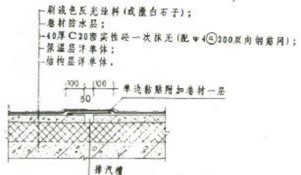
4 卷材屋排汽槽缝构造
