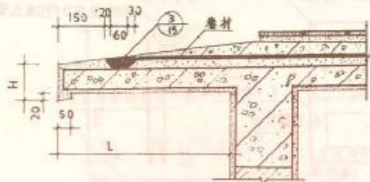
② 挑檐构造
