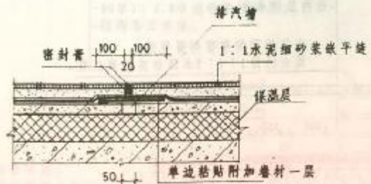
4 地砖面分格缝排汽槽构造
