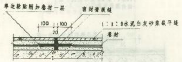
2 斗底砖面分格缝构造
