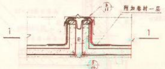
2 屋面檐沟变形缝
