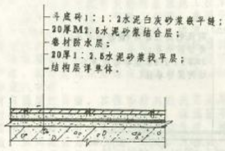
2a 2b 2c 斗底砖面上人屋面
