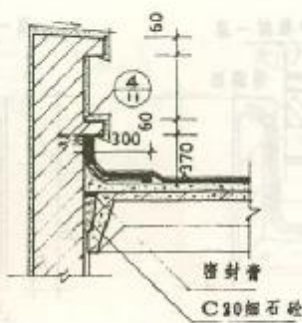
2 女儿墙泛水构造
