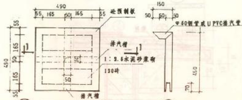
2 排汽槽平面
