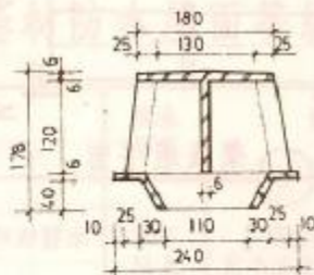
2 铸铁罩
