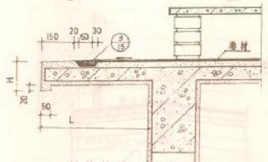
4 挑檐构造
