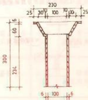
2 铸铁罩
