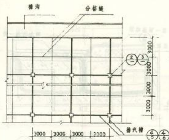
1 分格缝、排汽槽布置平面
