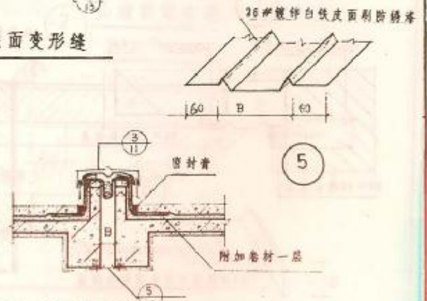
④ 屋面变形缝
