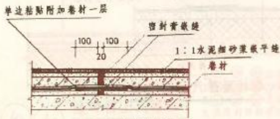
3 地砖面分格缝构造
