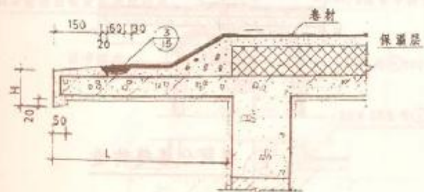
2 挑檐构造
