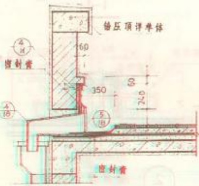
② 女儿墙外排水
