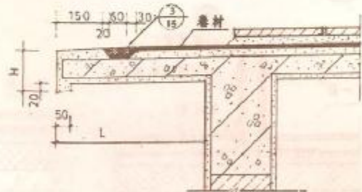
④ 挑檐构造
