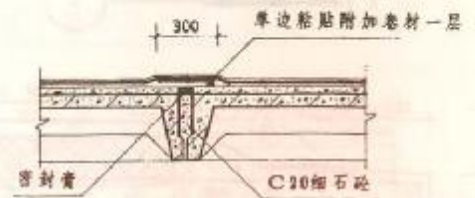
3 板间分格缝构造
