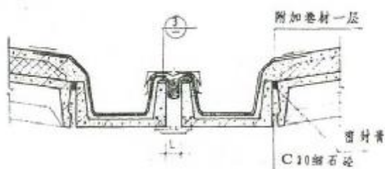
1 内天沟泛水构造
