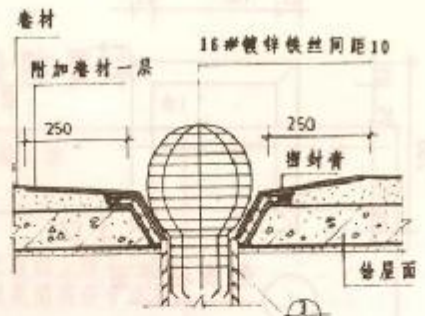
4 铅丝球罩
