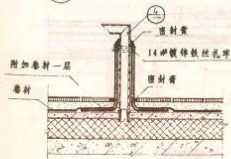
3 排汽管构造
