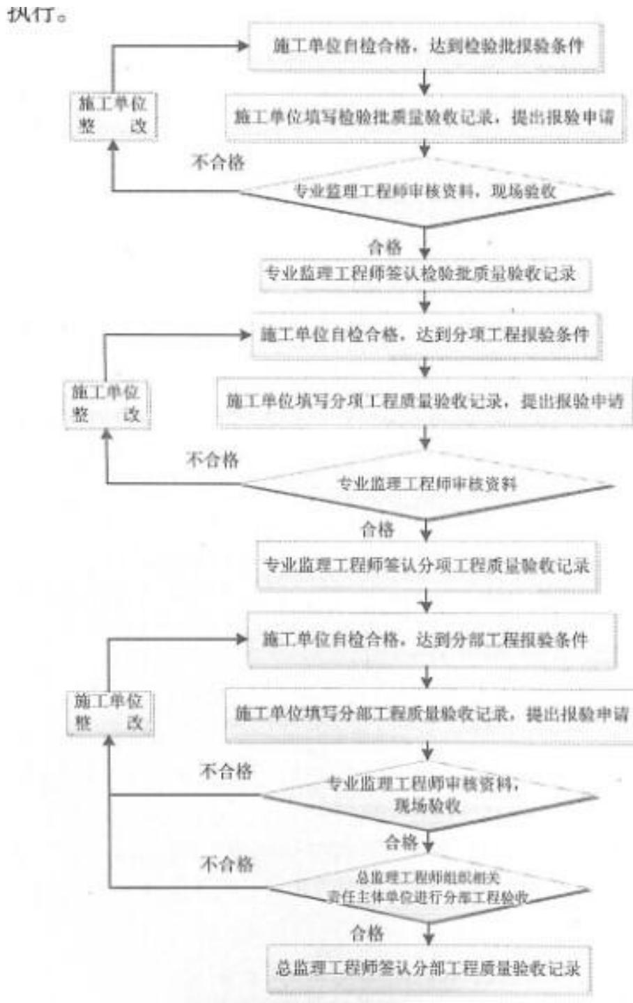
图 6.2.3 检验批、分项、分部工程验收程序
