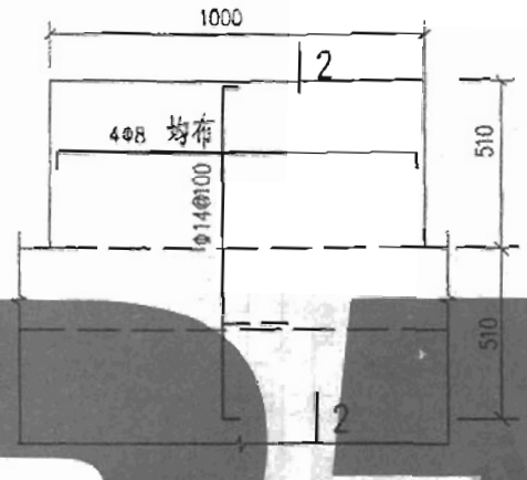
SWX-N2首层挑板配筋图 用于立面图三
