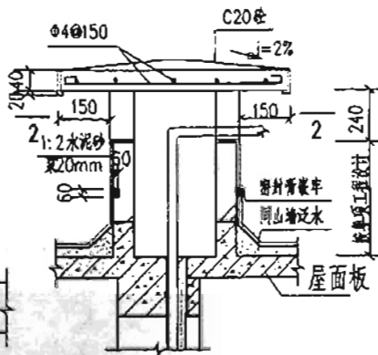
管窟出屋面做法
