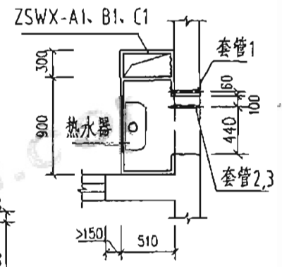
墙体预埋套管详图
