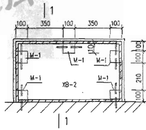
安装箱与墙体拉接
