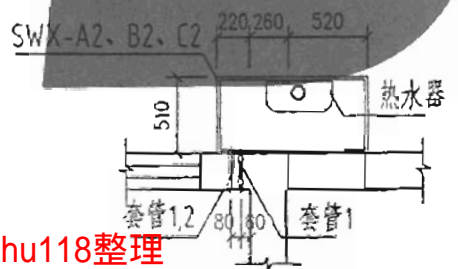
墙体预埋套管详图
