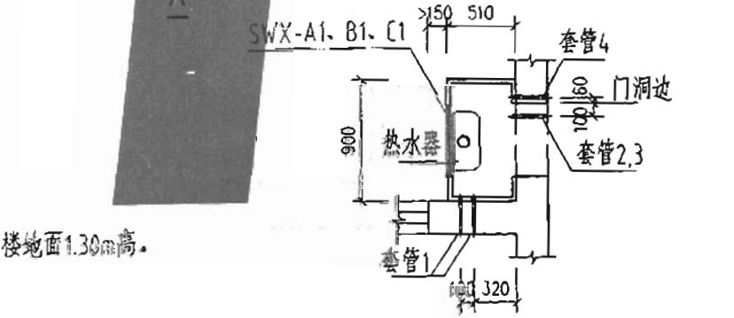
墙体预埋套管详图
