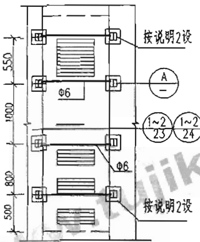
安装箱与墙体拉接
