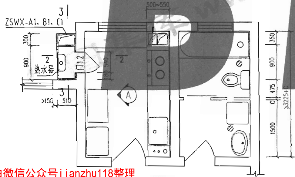
PM-3平面图
