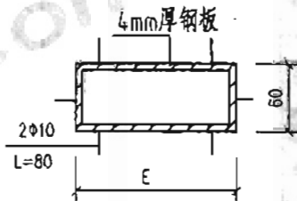
穿圈梁预埋方管平面图
