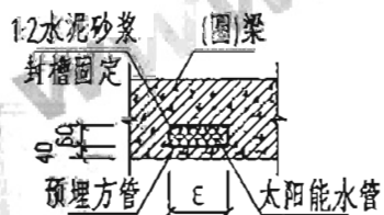
管窟出屋面做法
