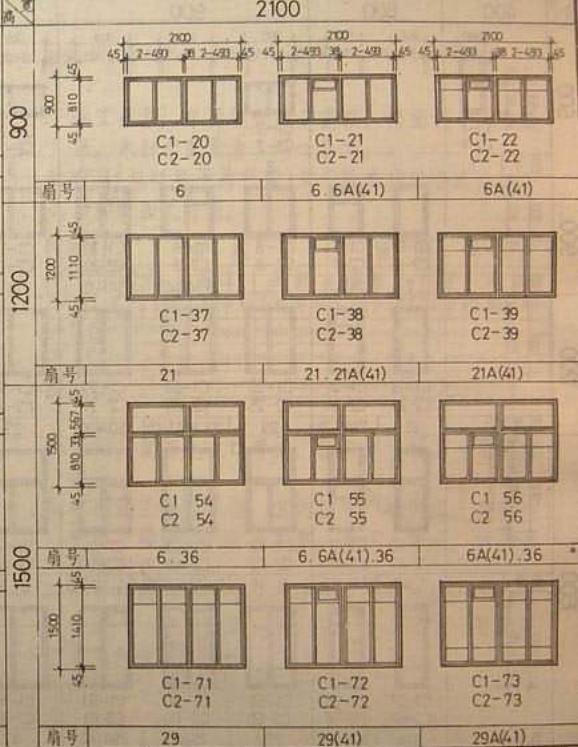
C1、C2平开窗立面图(二)
