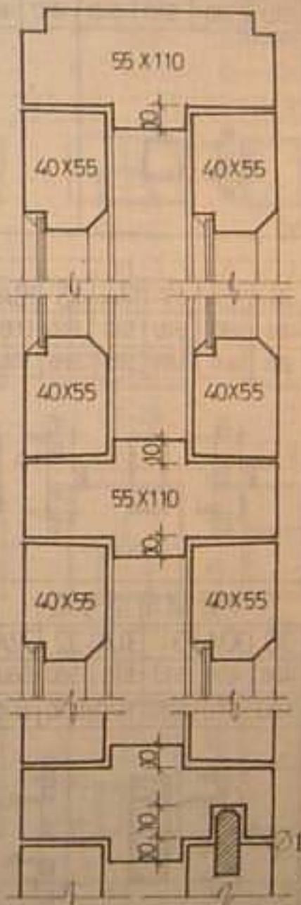
C2双层平开窗节点详图
