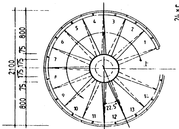
C型 1-1 平面
