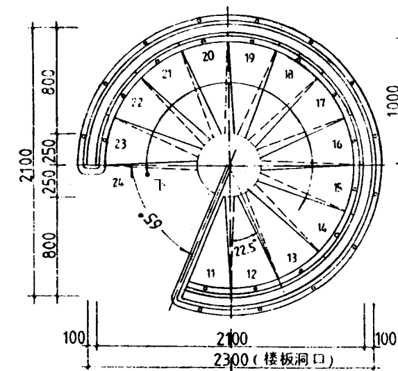
C型 2-2 平面
