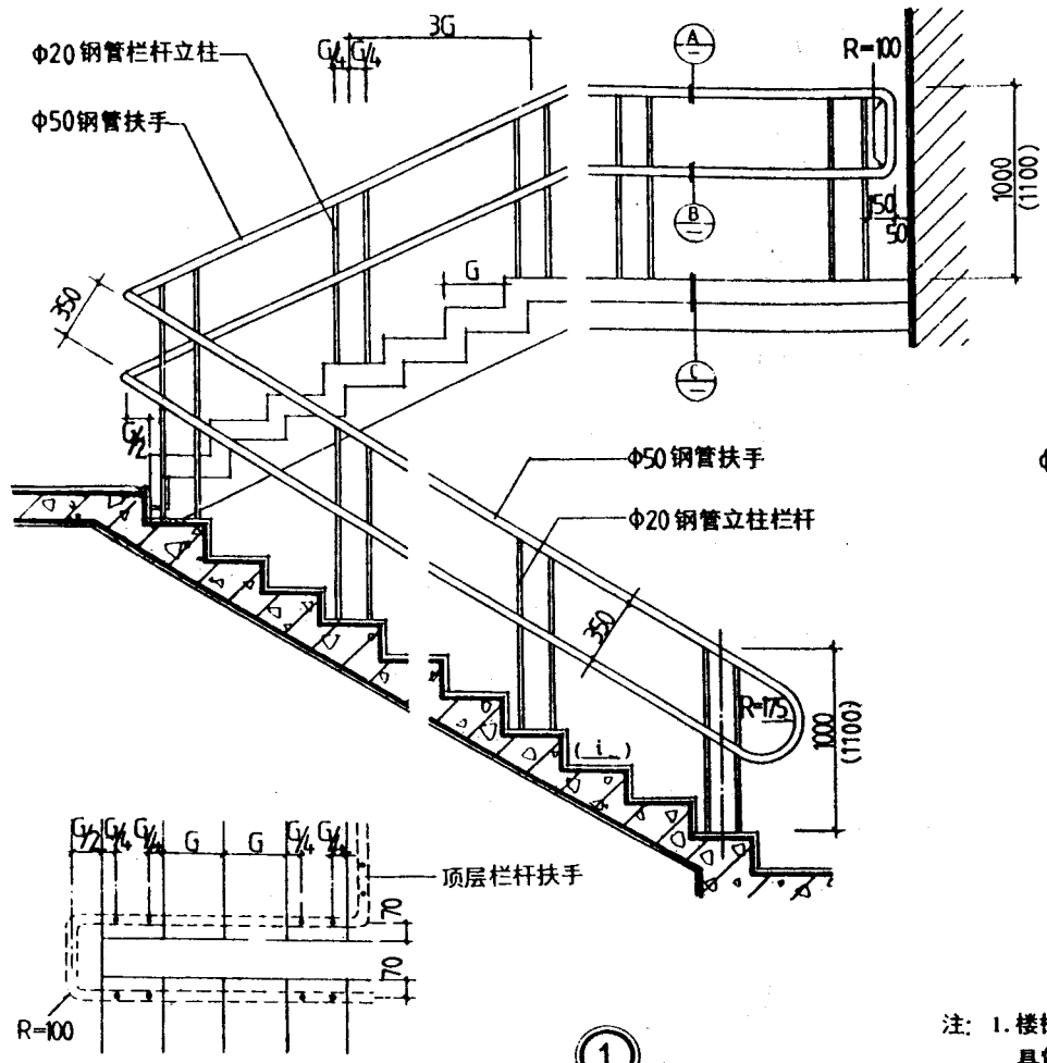
栏杆立柱平面示意
