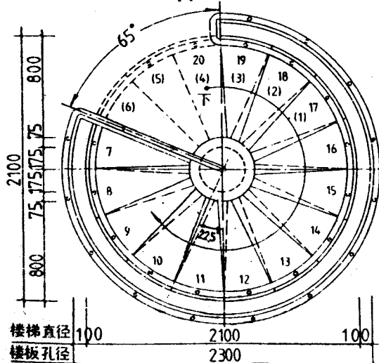
B 型平面
