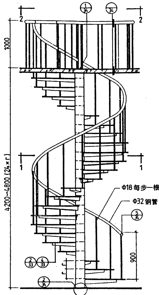
D型立面
