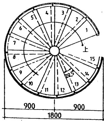
D型1-1平面
