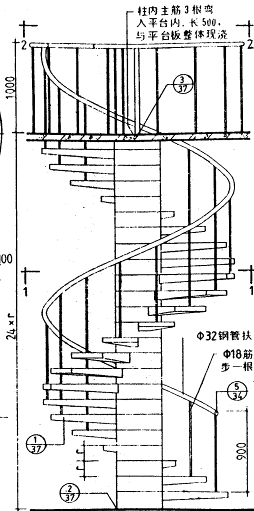
C型立面
