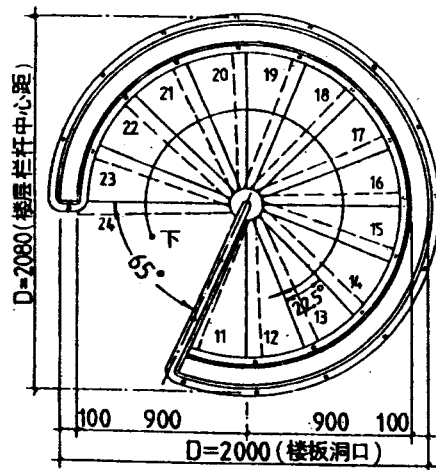
D型2-2平面
