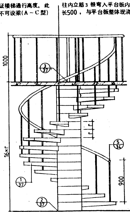
A 型立面
