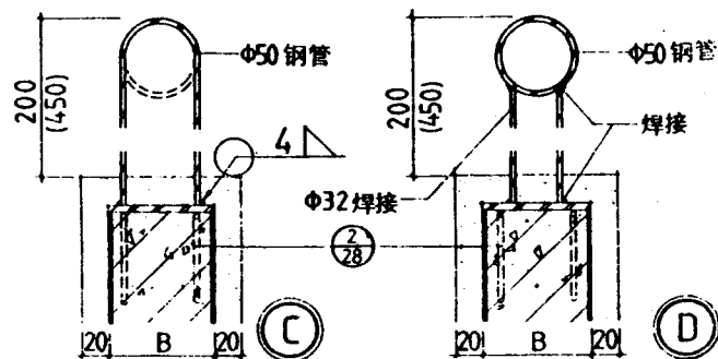
注：1. 金属栏杆的油漆、水刷石石子、涂料的品种、规格、颜色由设计人定 2. 栏板厚 B = 80 ，或按工程设计。
