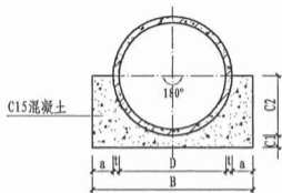
基础断面图
