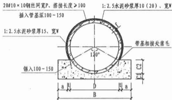
接口横断面
