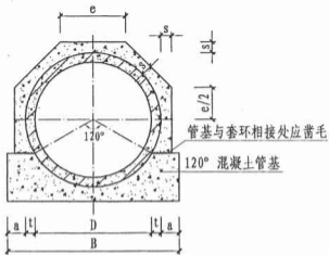
接口横断面
