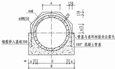
接口横断面
