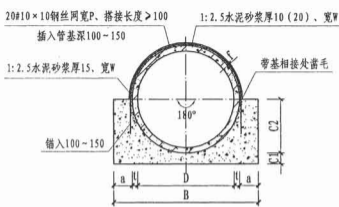
接口横断面
