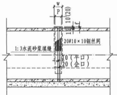
接口纵断面
