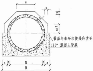
接口横断面
