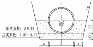
基础断面图
