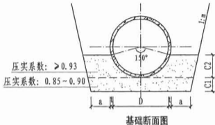
基础断面图
