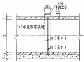
接口纵断面
