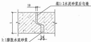
接口纵断面
