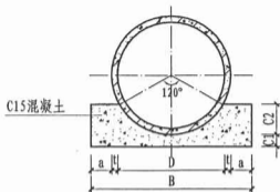
基础断面图
