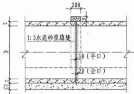
接口纵断面
