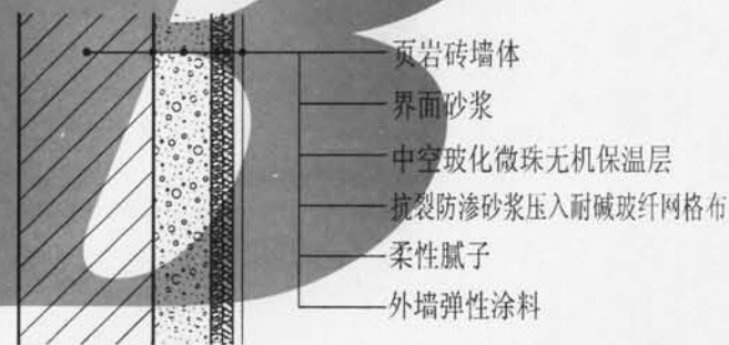
中空玻化微珠页岩砖外墙外保温隔热体系
