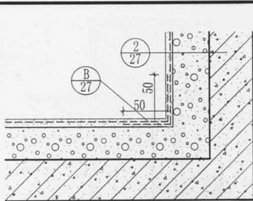
① 外墙阴角
