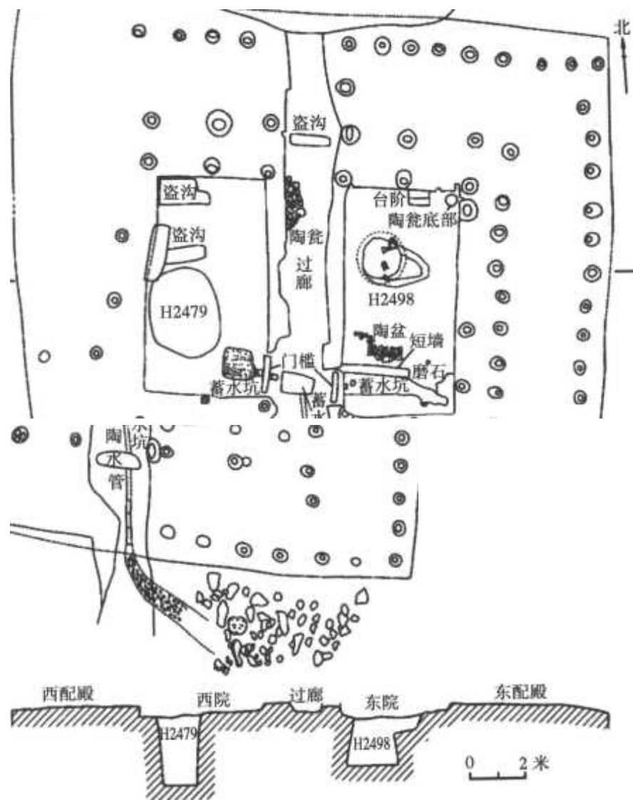
F79平面及剖面图
