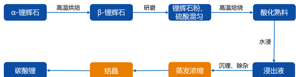
图表 18: 硫酸锂生产工艺流程
