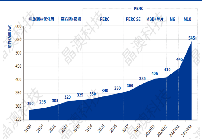
图表 52：通过多维技术持续提高组件功率
