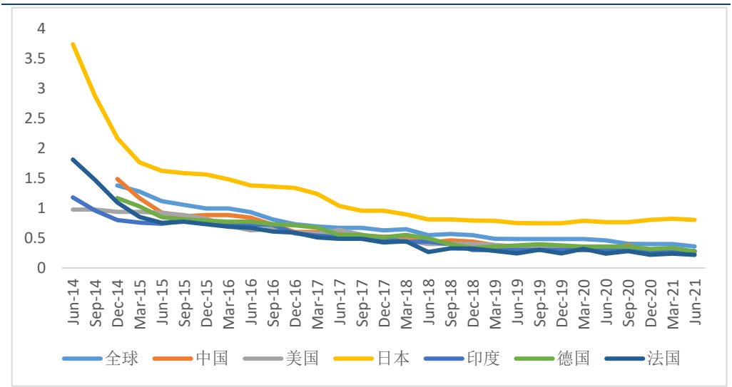
图表 15: 光伏 LCOE 大幅下降，经济性优势逐渐凸显
