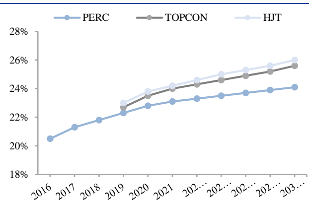
图表 45：不同类型的电池转换效率
