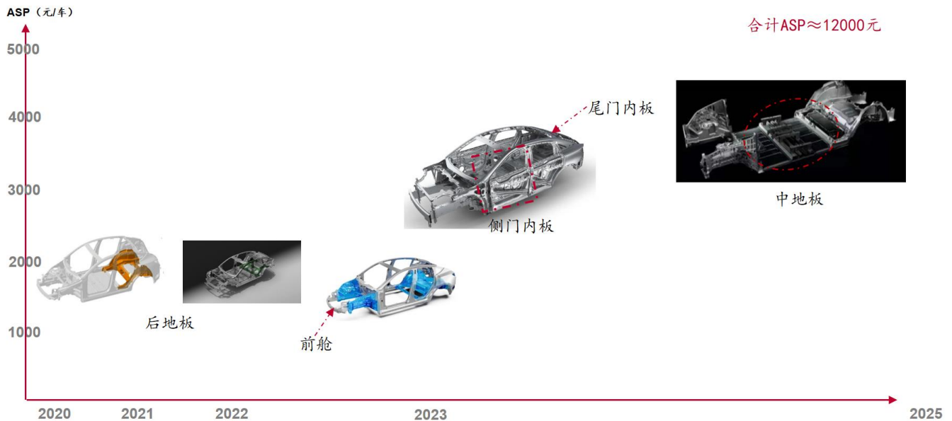
图表 18：一体化压铸应用范围、ASP 与预计量产时间
