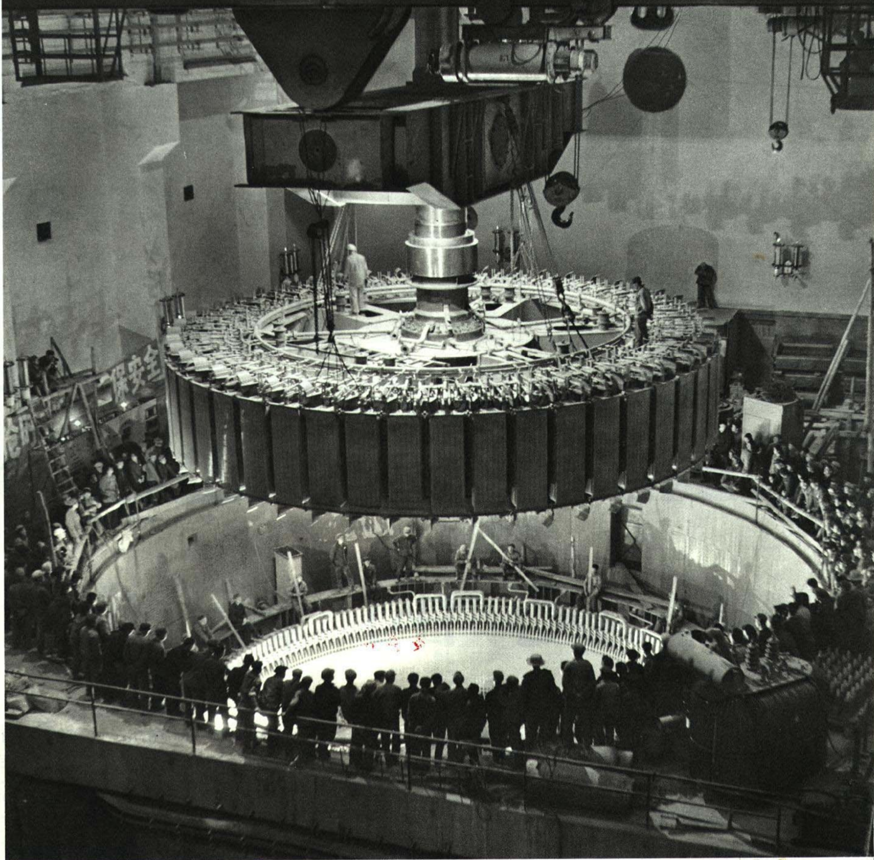
安装国产大型水轮发电机组的转子。
