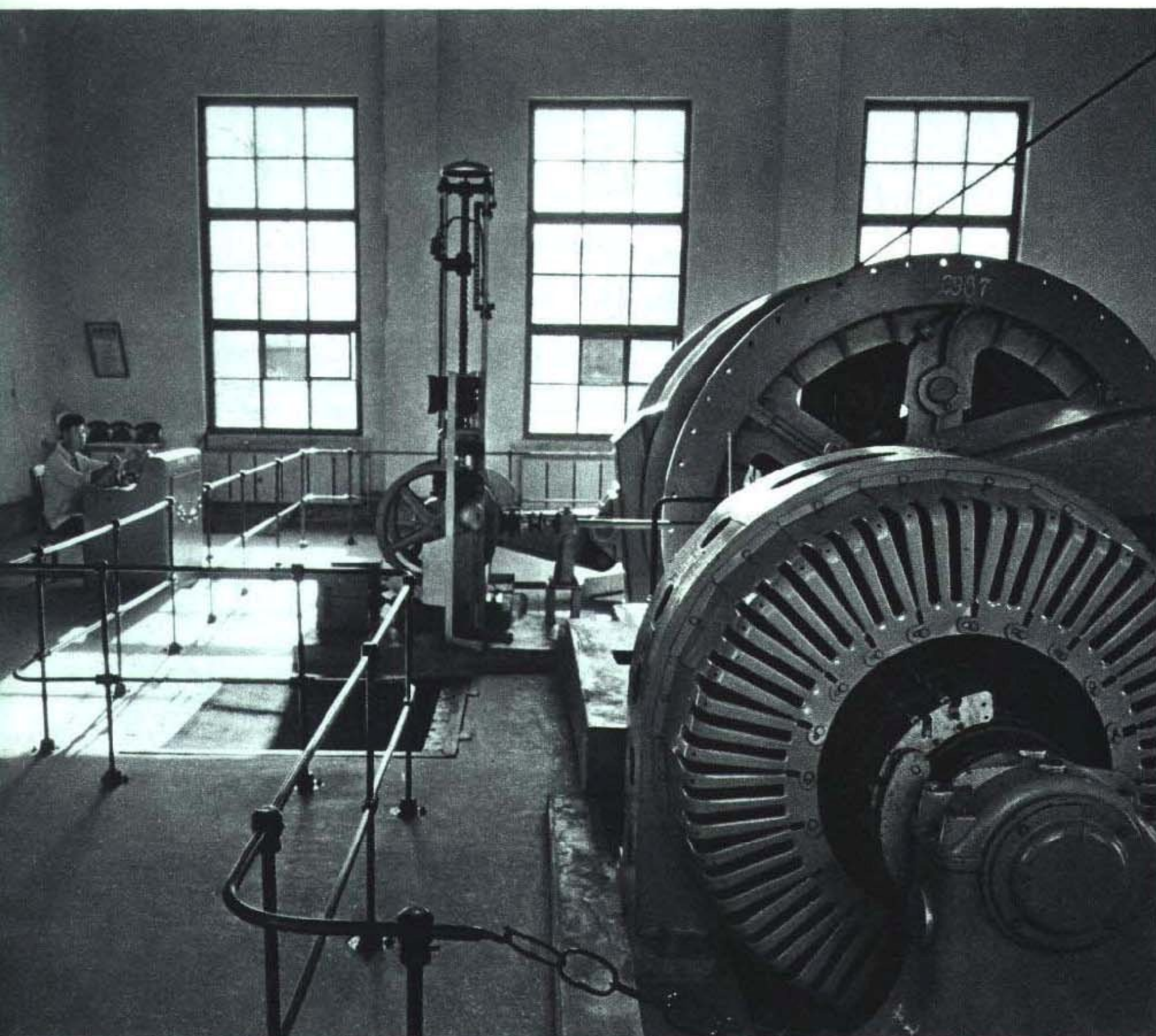
张新竖井的提升机室
