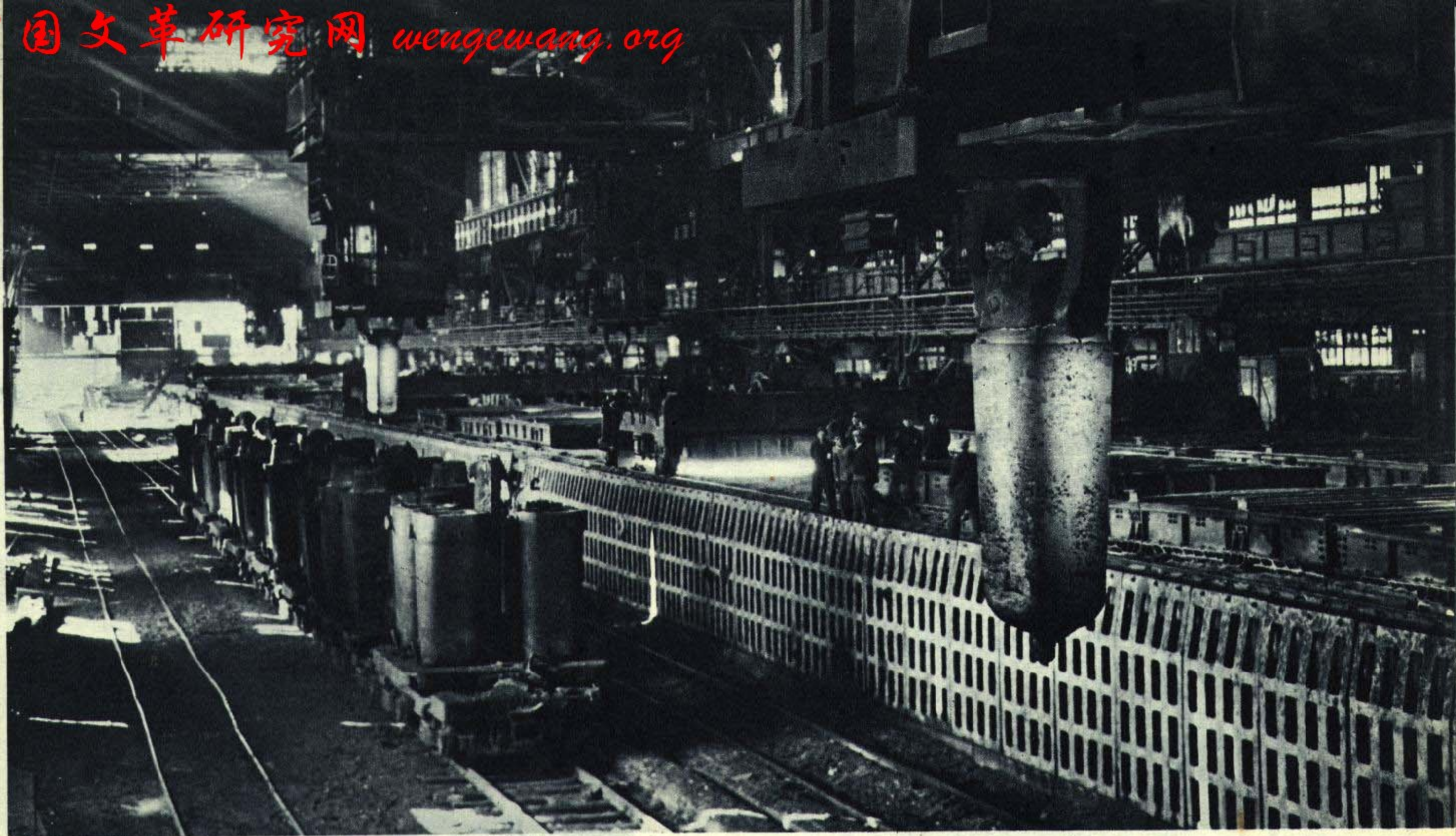
送往初轧厂的大钢锭
