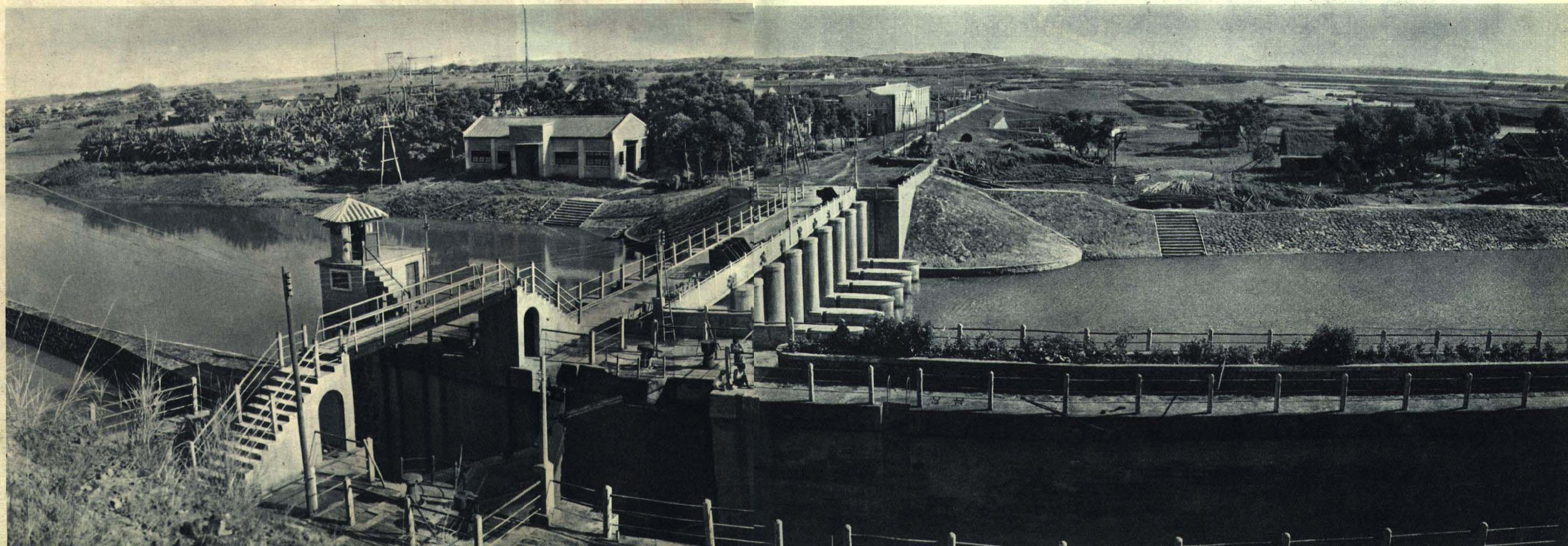
南海县樵北大围电力排水站
