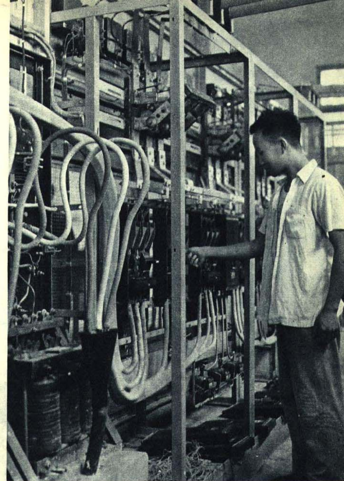
中山县庙涌电力排水站的设备
