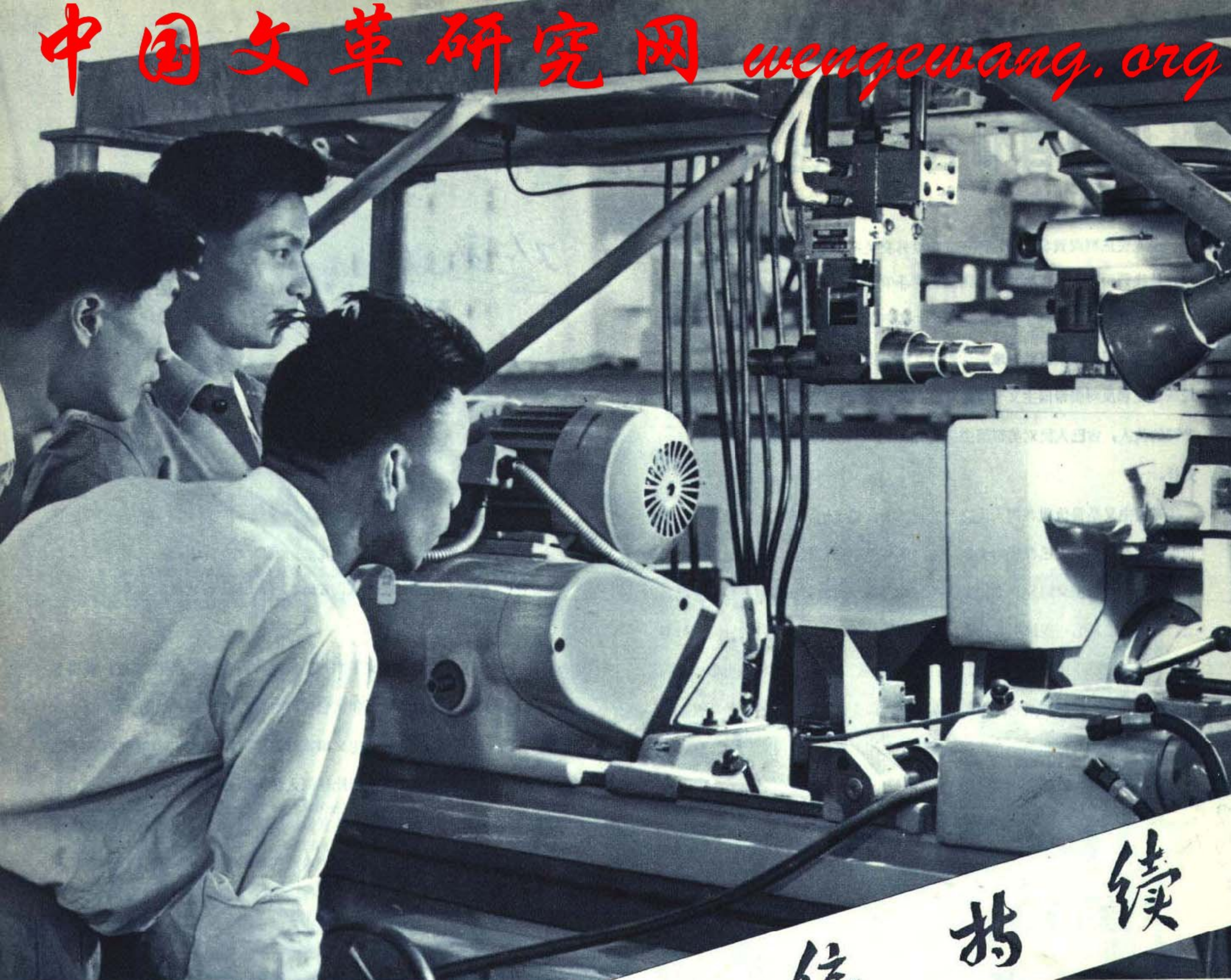
上海机床厂工人试制成功的200毫米自动外圆磨床。这是机械手正在自动送料
