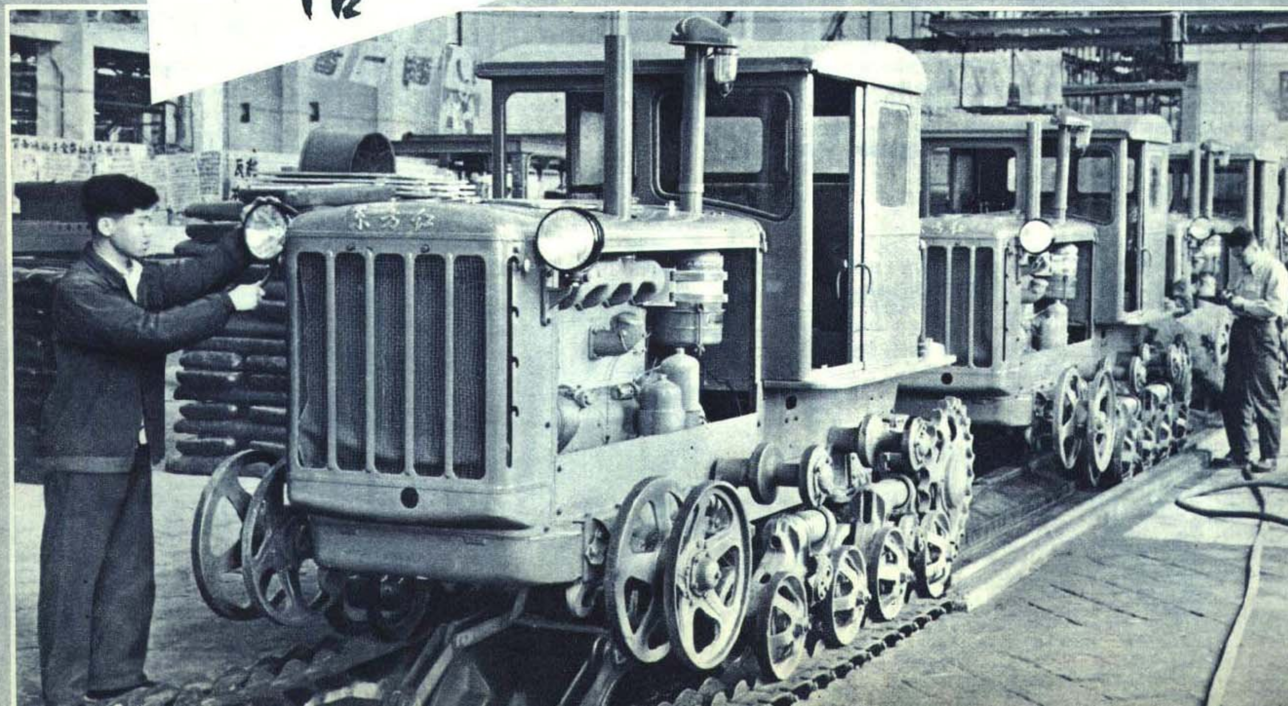
洛阳拖拉机厂职工为了支援农业，大闹技术革新。总装配线的工人连续攻破五个关键，使装车速度比原来加快了将近一倍 杨震河摄影
