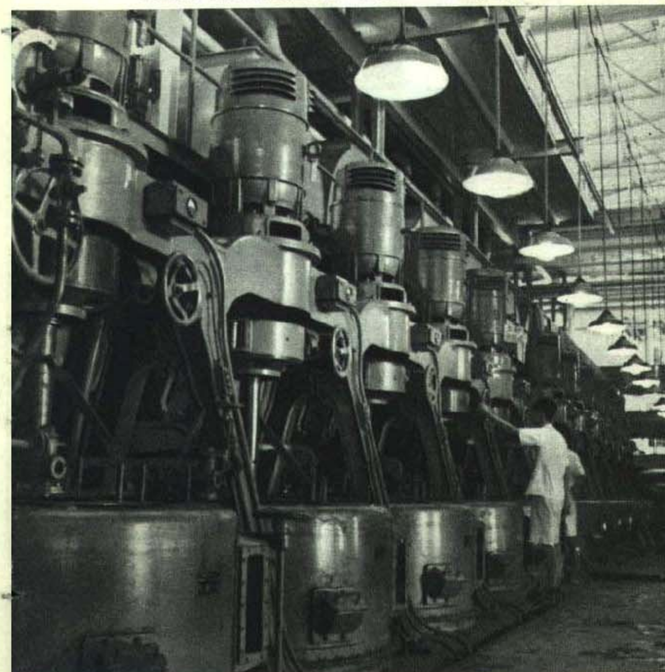
佳木斯友谊糖厂的分离设备。这个厂已在去年12月投入生产，它是中波友谊的又一结晶。 胡侑摄影
