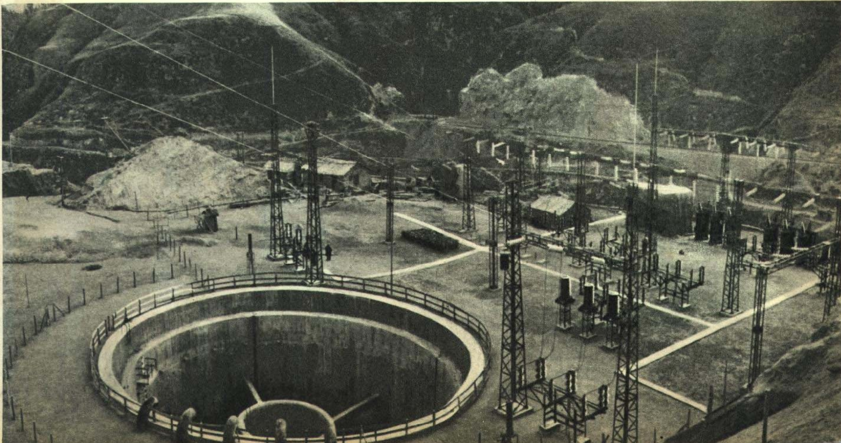
變電所和調壓井
