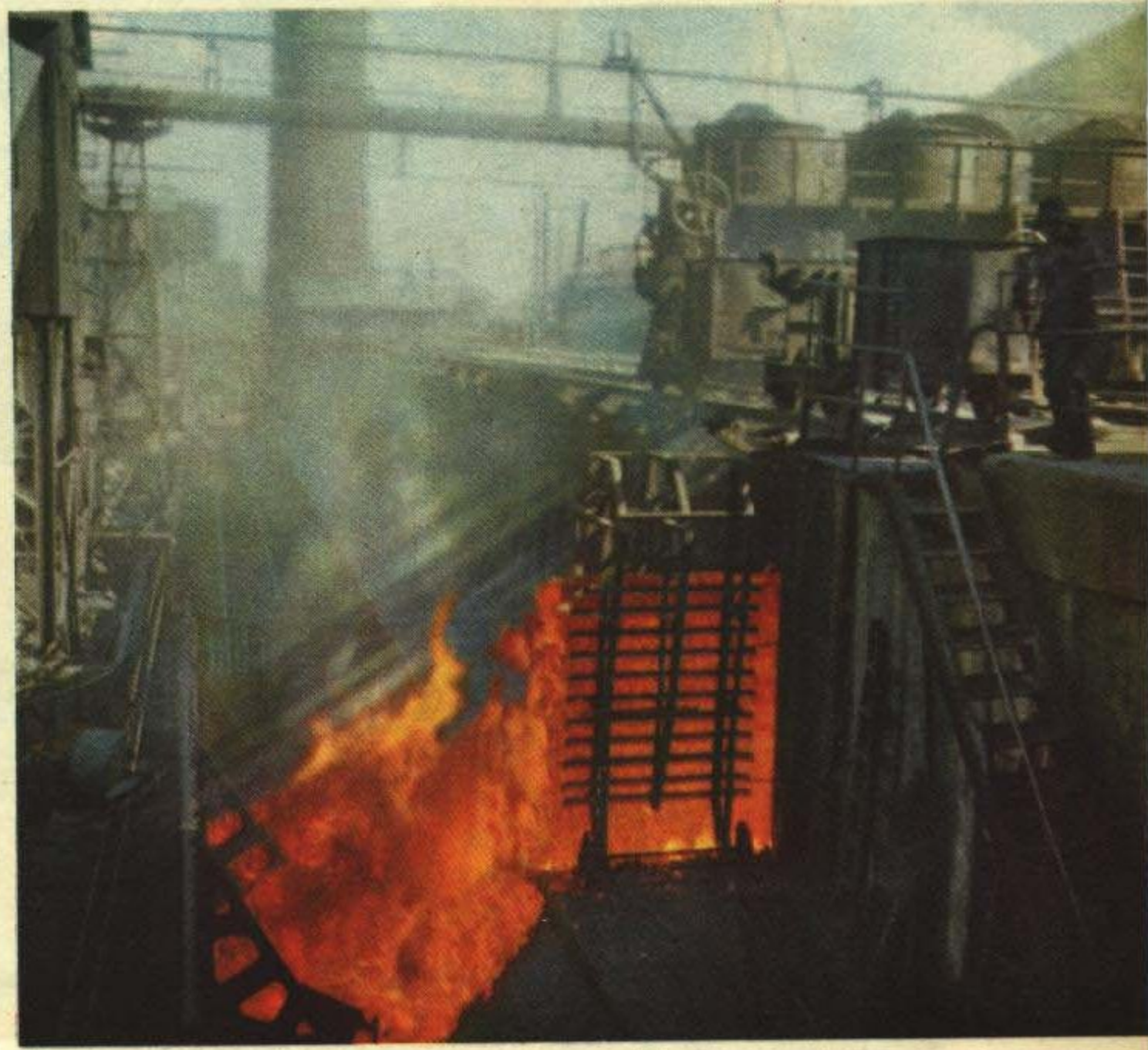
煉焦爐煉出來的焦炭，經過消火後，就可以運到本溪煉鐵廠和馬鞍山等地做為煉鐵的燃料。
