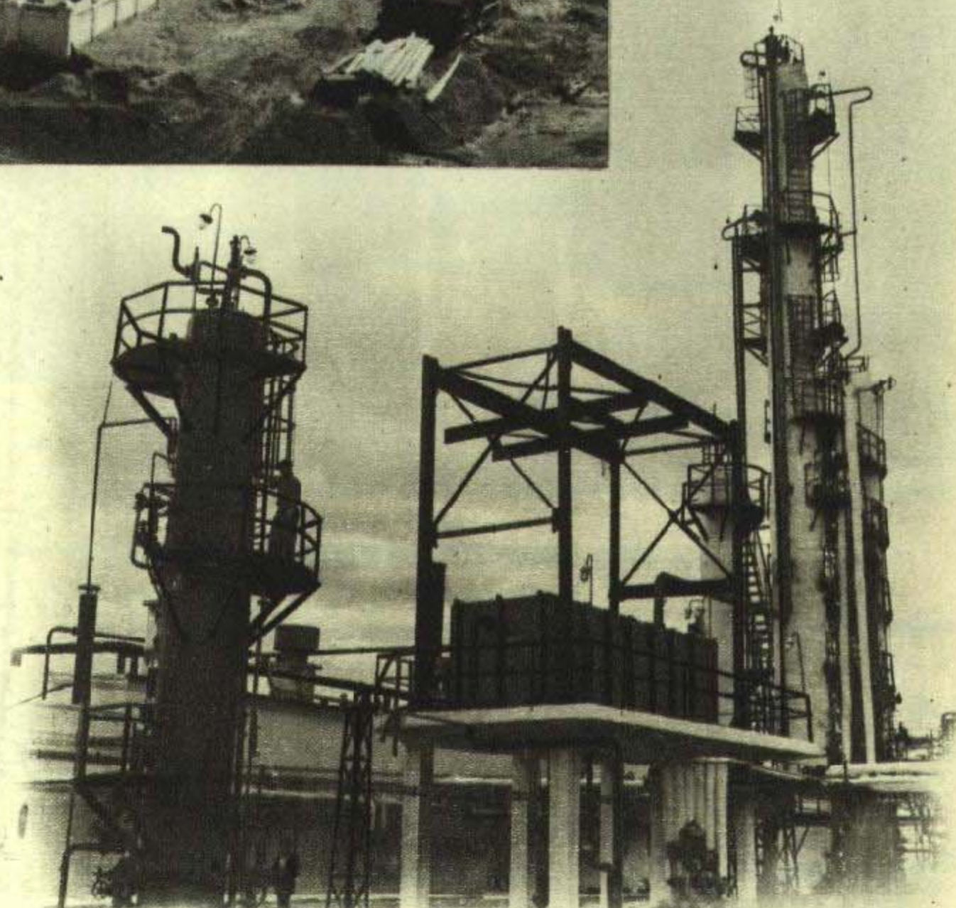
中蘇石油公司用蘇聯最新的設備建成的自動化煉化廠，可以從柴油和原油中提煉汽油。
