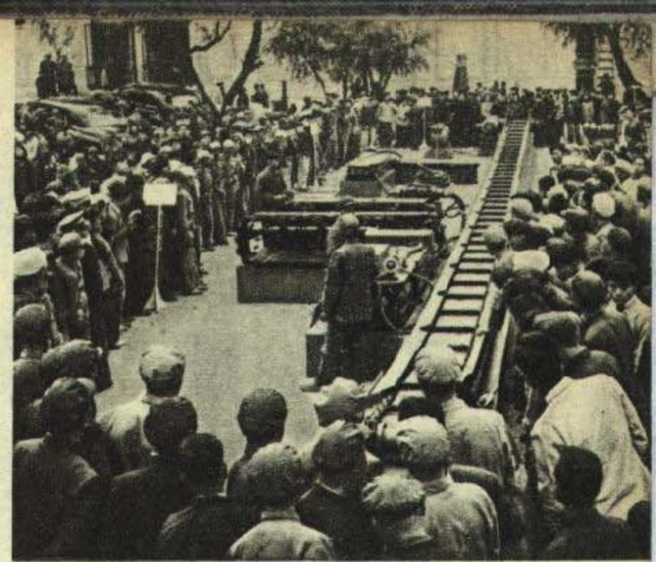
把採煤的主要過程全部自動化的“頓巴斯”採煤聯合機，每小時可採煤五十到一百一十噸。
