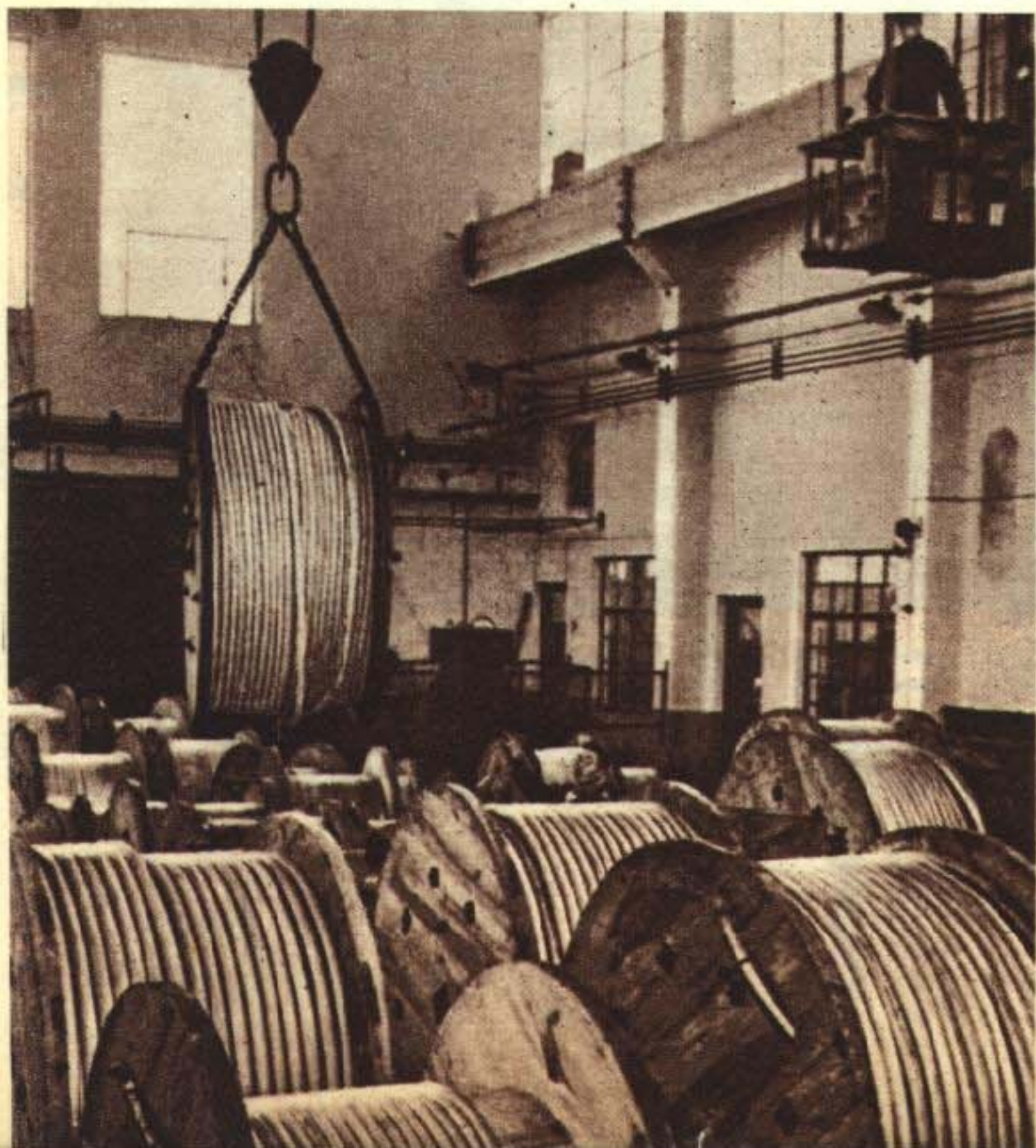
上海各重工業工廠的工人大力支援國家基本建設 上海市各重工業工廠，經過三年來的恢復與發展，已從過去僅能修理裝配機械零件的工廠發展到能够生產各種發電機、鍋爐、電動吊車及精密工具等的工廠了。當國家大規模經濟建設開始後，上海市國營和私營重工業工廠的工人都積極生產，製造了大批產品，支援全國的基本建設。左圖：上海電綫廠工人製造的大批粗電綫；右圖：上海虬江機器廠製成的大批新式內圓磨床。
