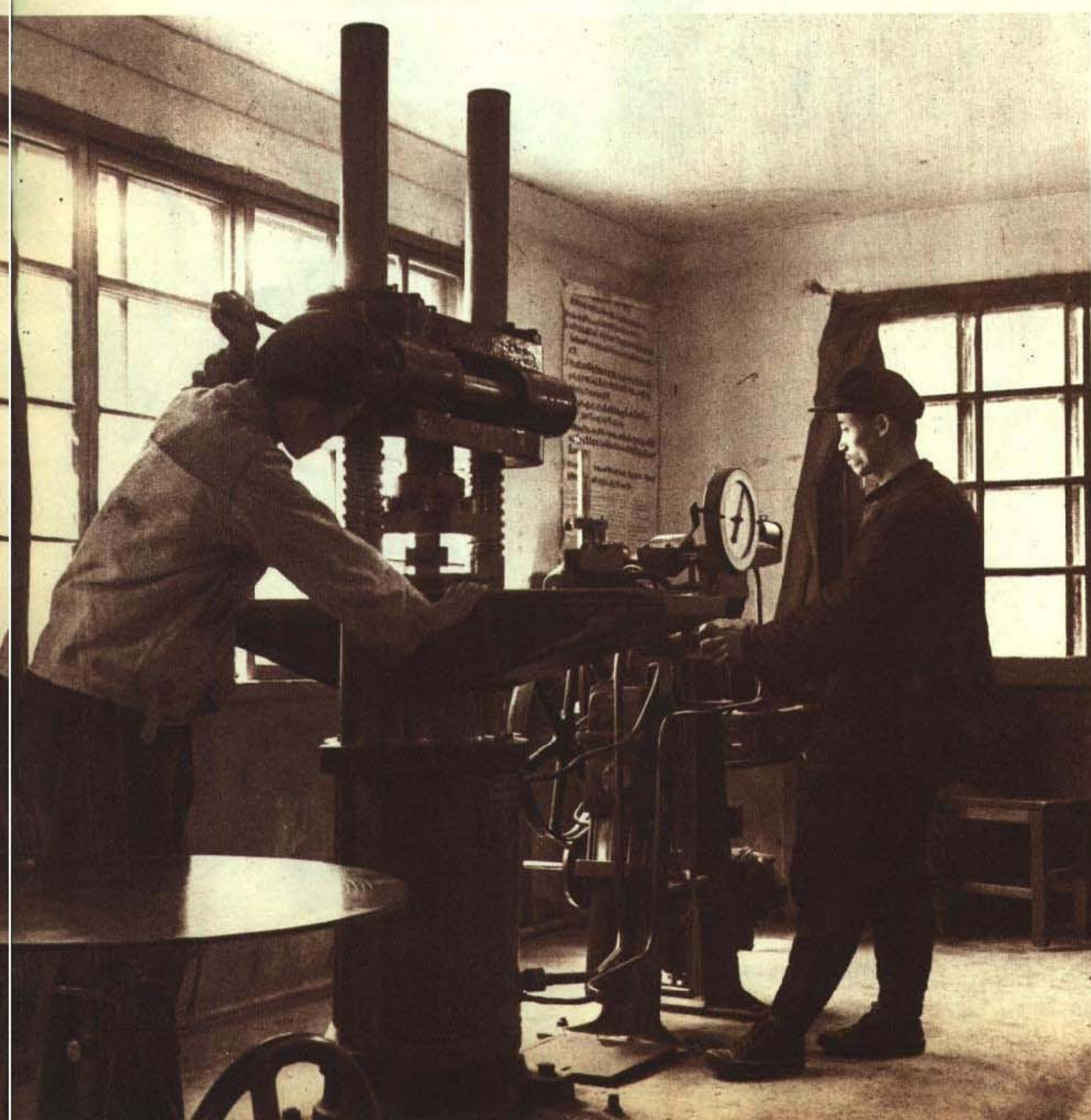
化驗室的劉恩奎小組在油壓機上試驗混合水泥“試塊”的耐壓力。通過這種試驗來保證混合水泥的質量。
