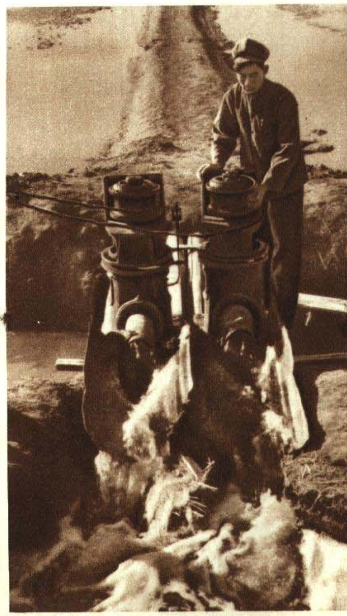
在各段導水溝上工作的電動揚水機。（在從前沒有電氣化的時候，一般地用水車或風車抽水，效率很低；也有用柴油抽水機的，但燃料最貴，影響成本。）
